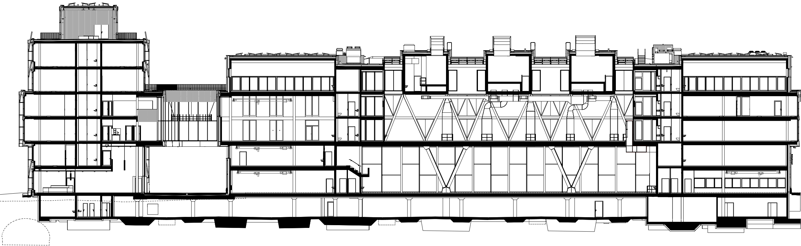
SCHNITT 9-9 HQ/TC
