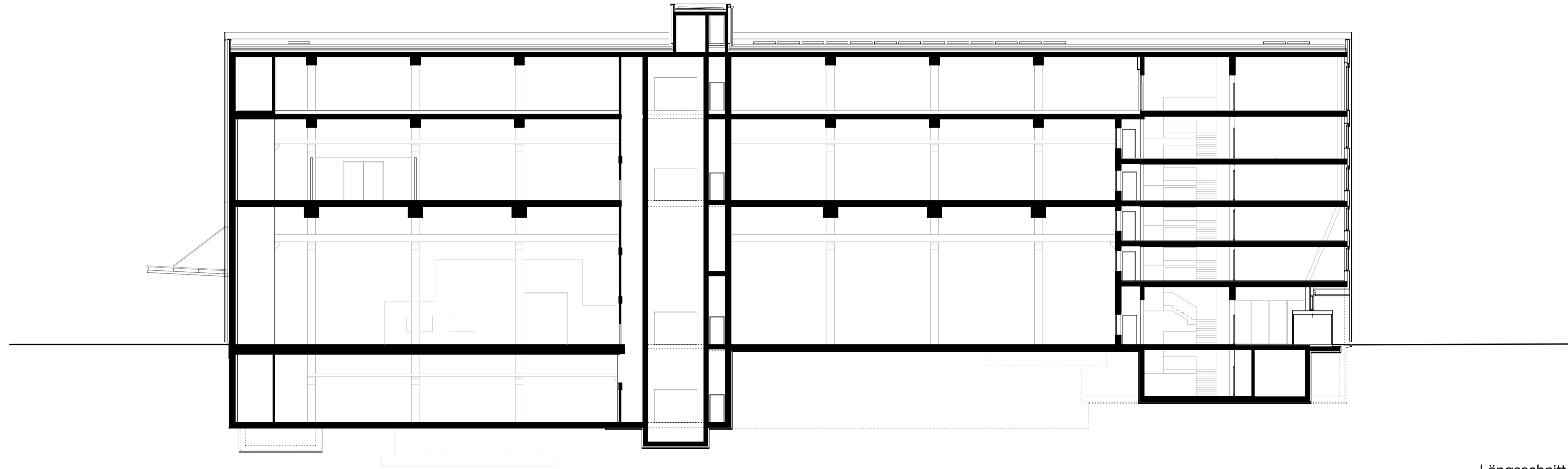
Längsschnitt A
