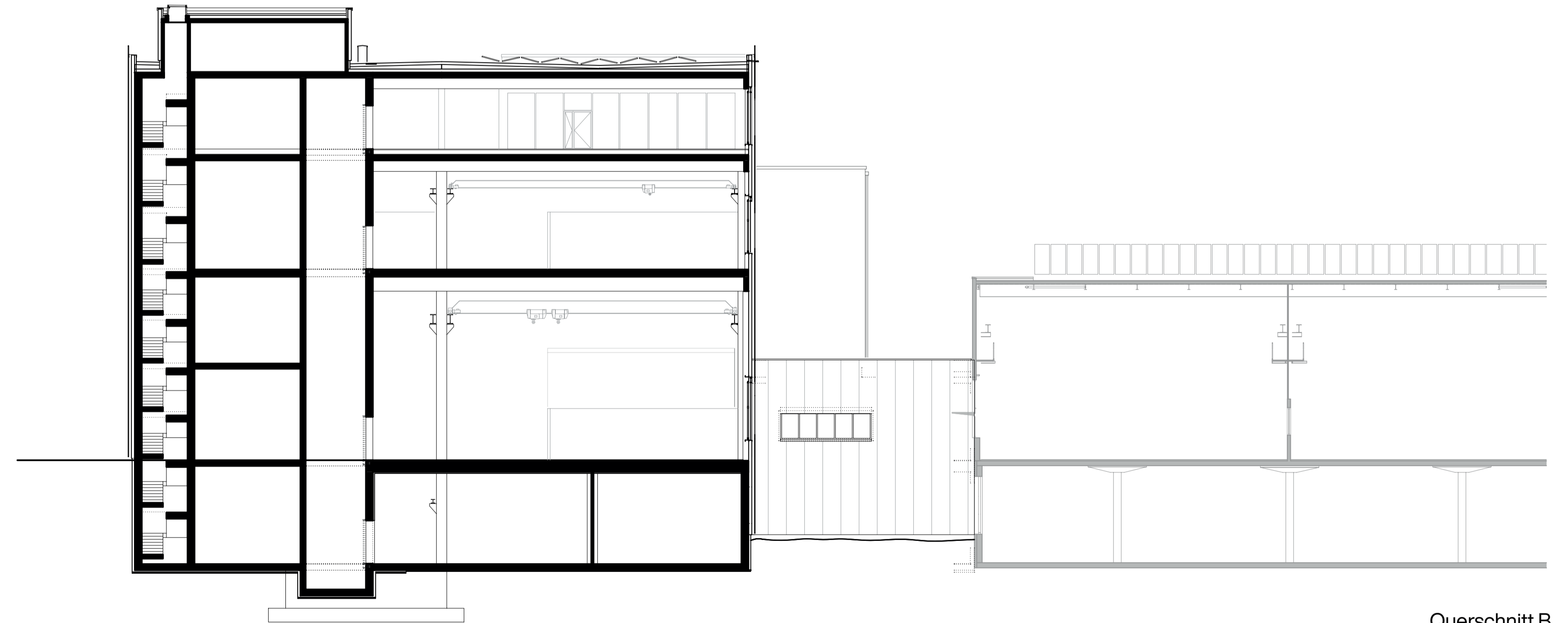
Querschnitt B
