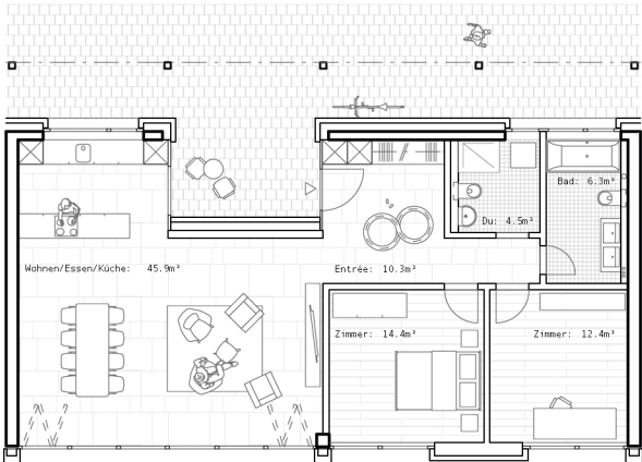
Geschosswohnung 3½ 94.1 m²
