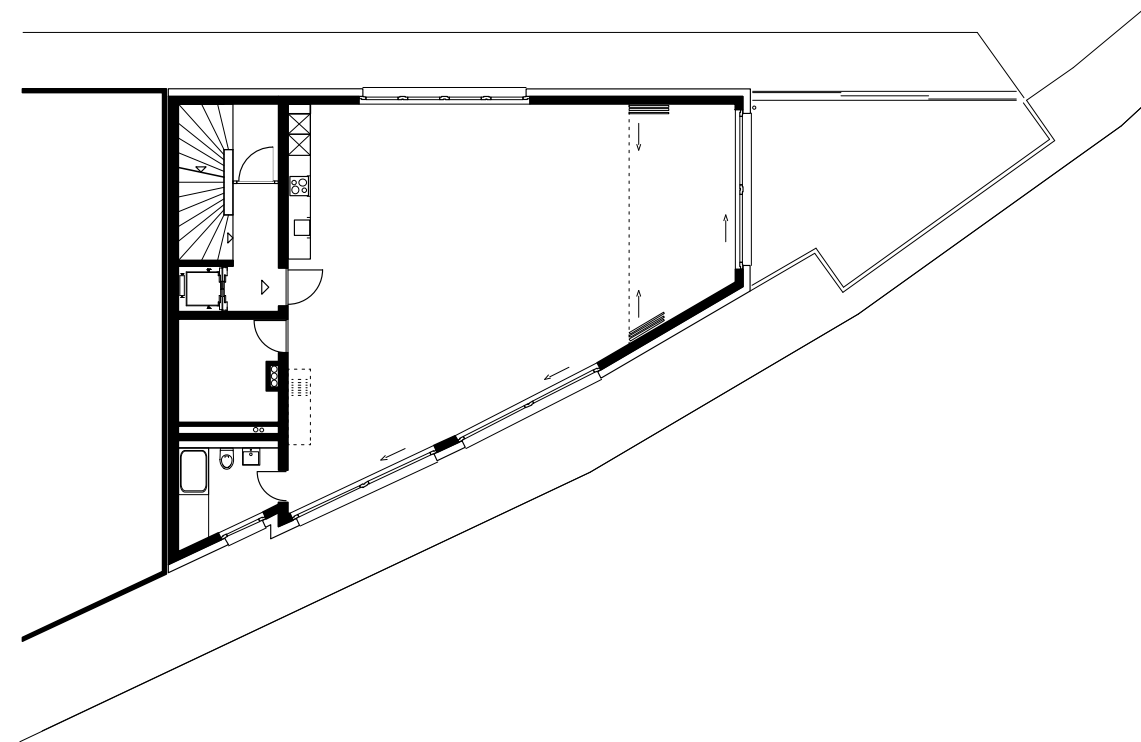
2.Obergeschoss
