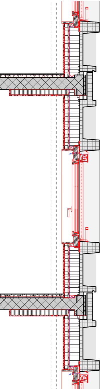
SCHNITT Mst. 1:33
