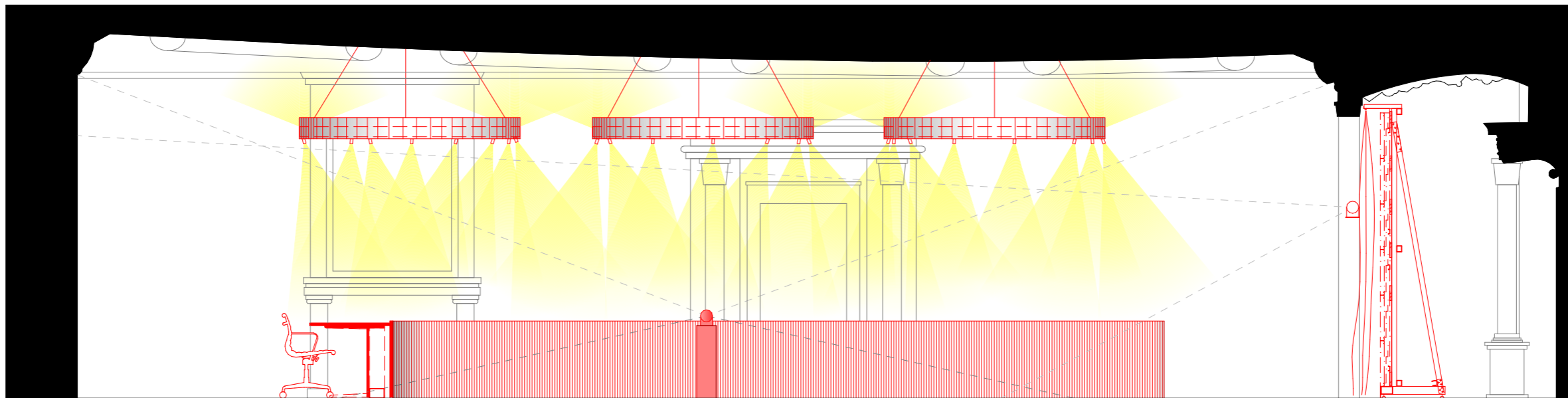
Längsschnitt Saal | 2. Obergeschoss
