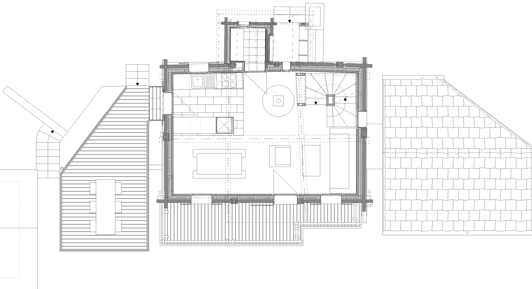
PLAN DU PREMIER ETAGE
