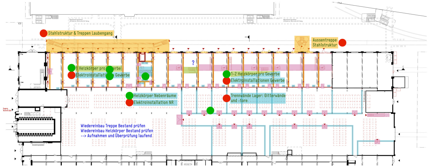
Grundriss EG
