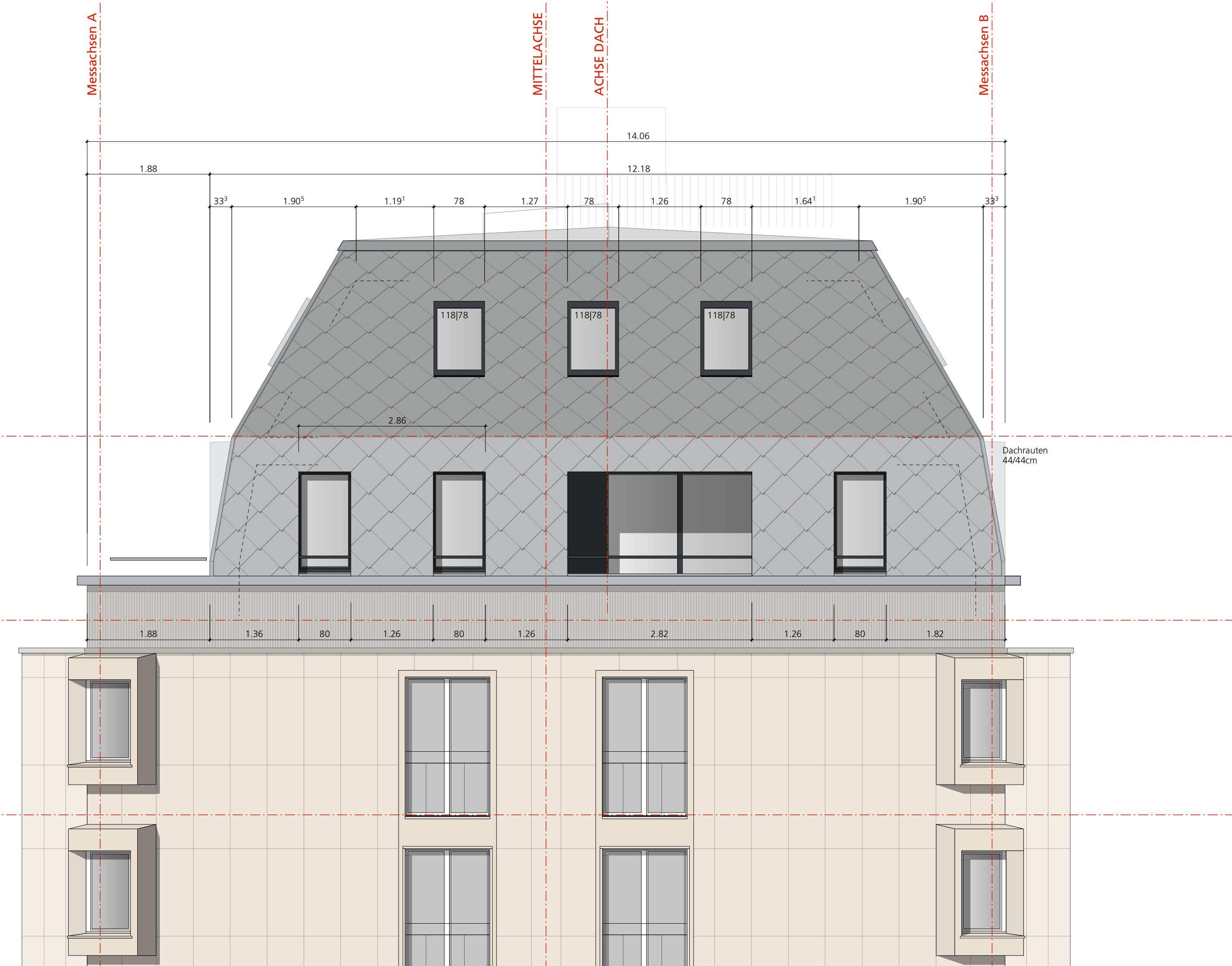
Nord-Ost Ansicht
