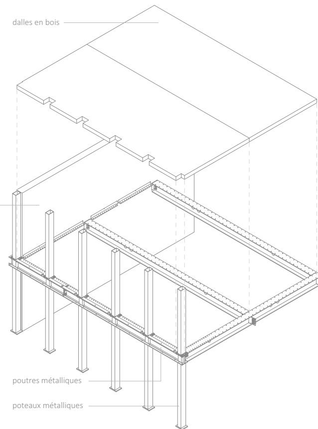
Détail de la structure mixte du bâtiment
