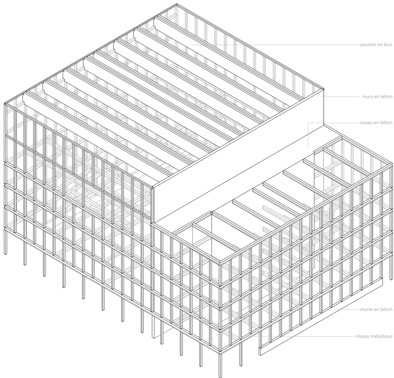
Axonométrie de la structure mixte du bâtiment
