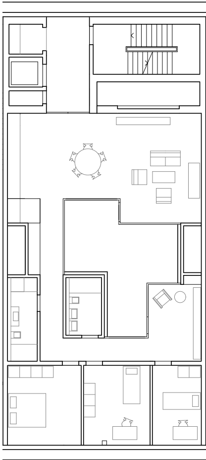
4. OG Geschosswohnung
