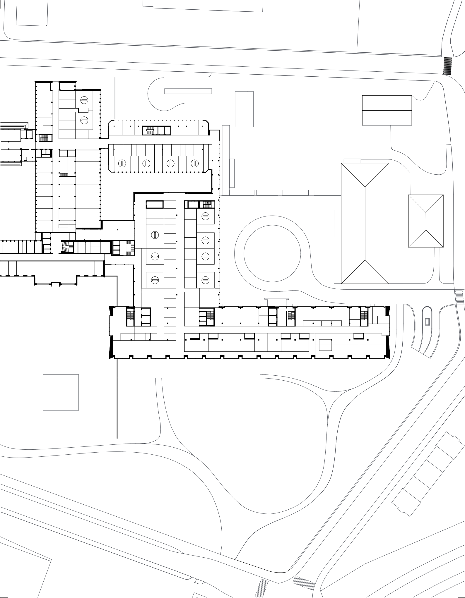
Grundrissplan 5. Obergeschoss
