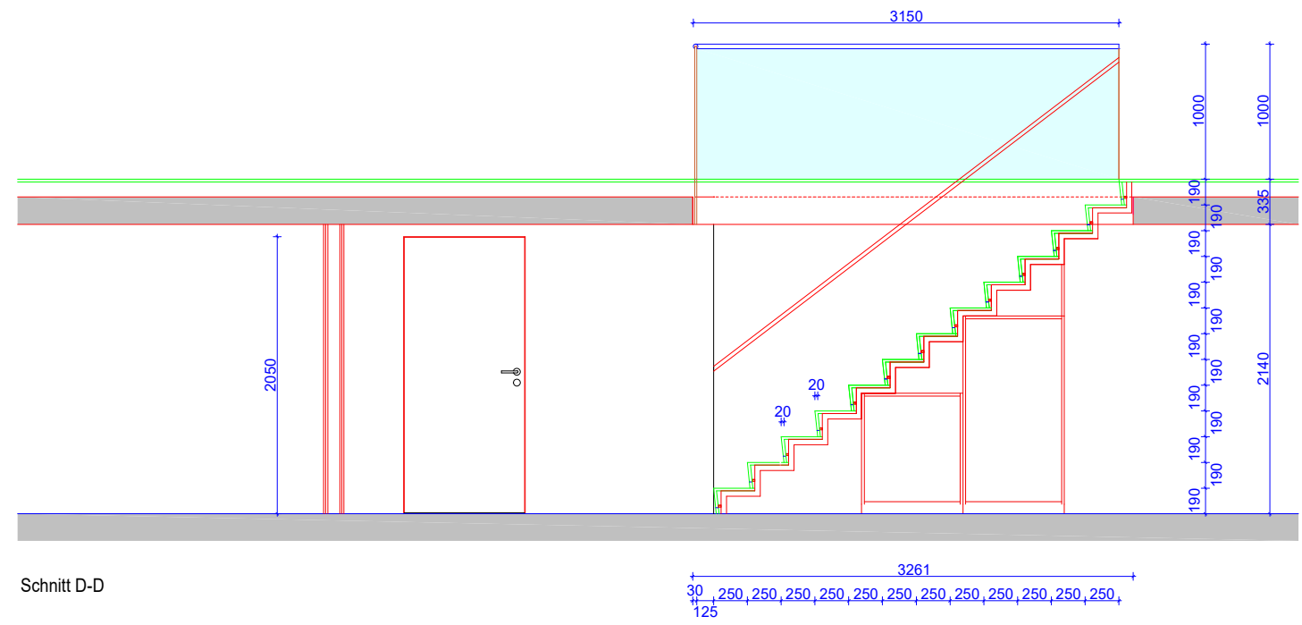
Schnitt D-D
