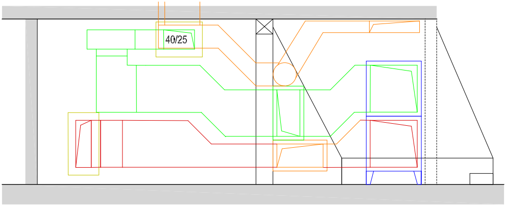
Schnitt G-G
