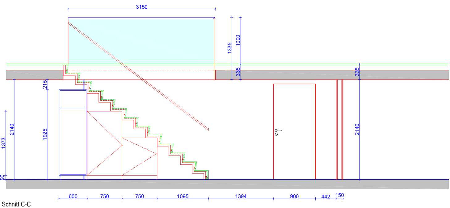
Schnitt C-C
