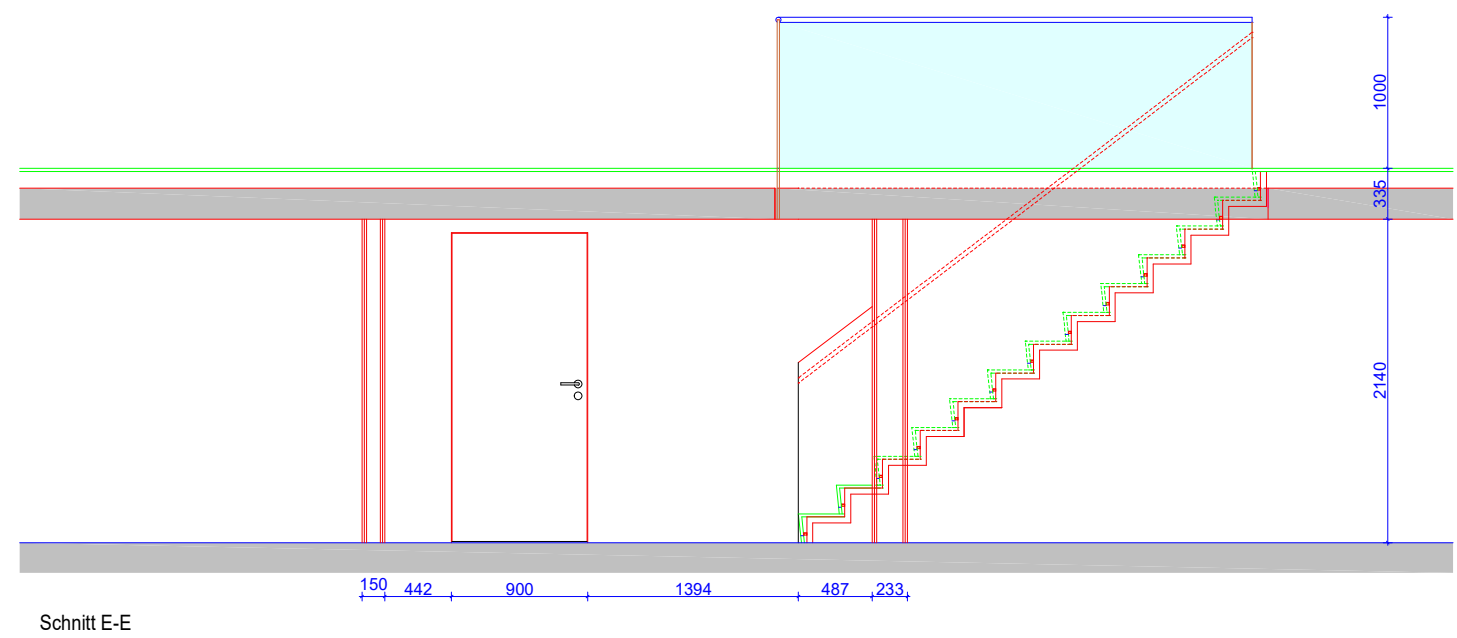
Schnitt E-E
