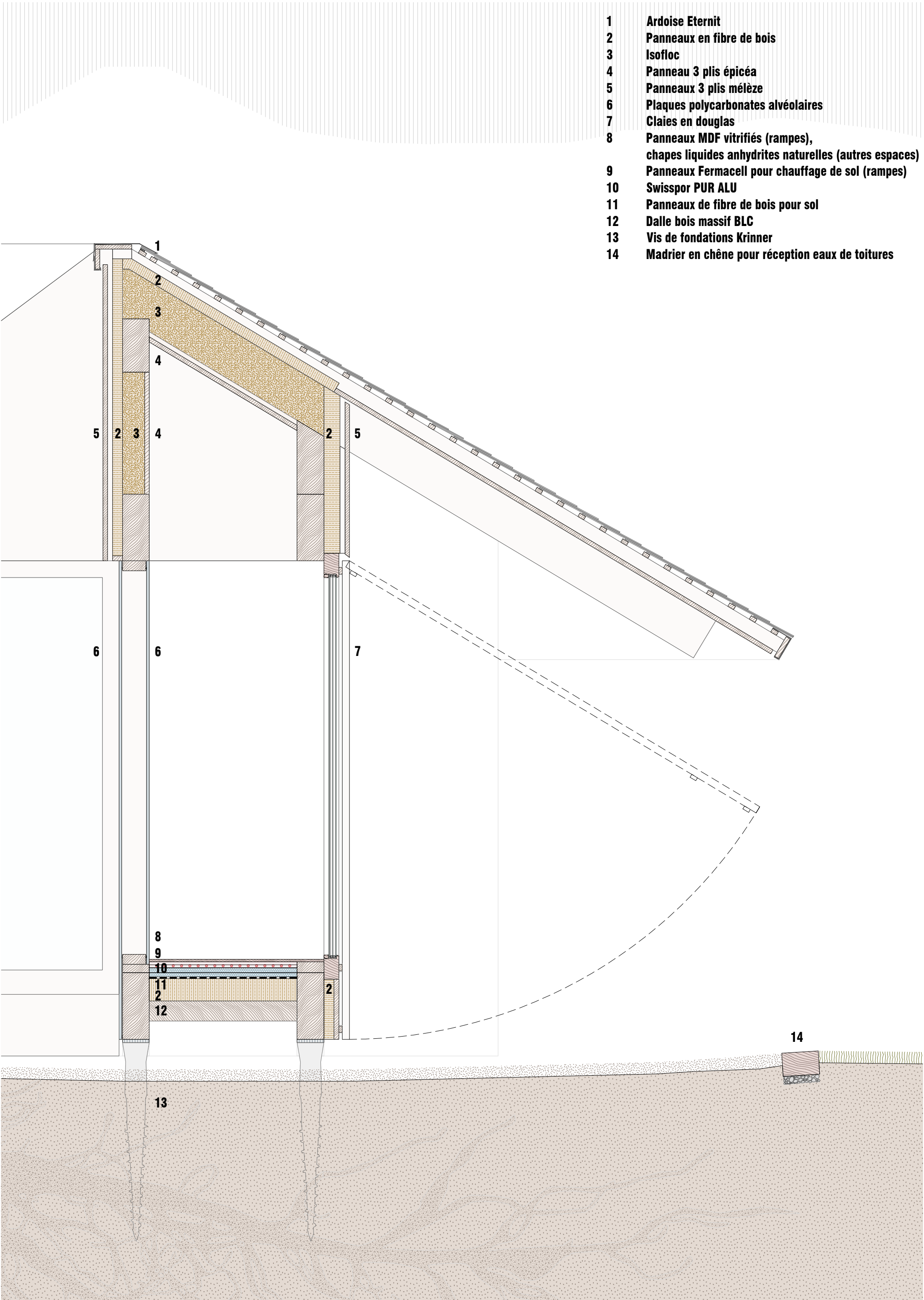
Coupe détail
