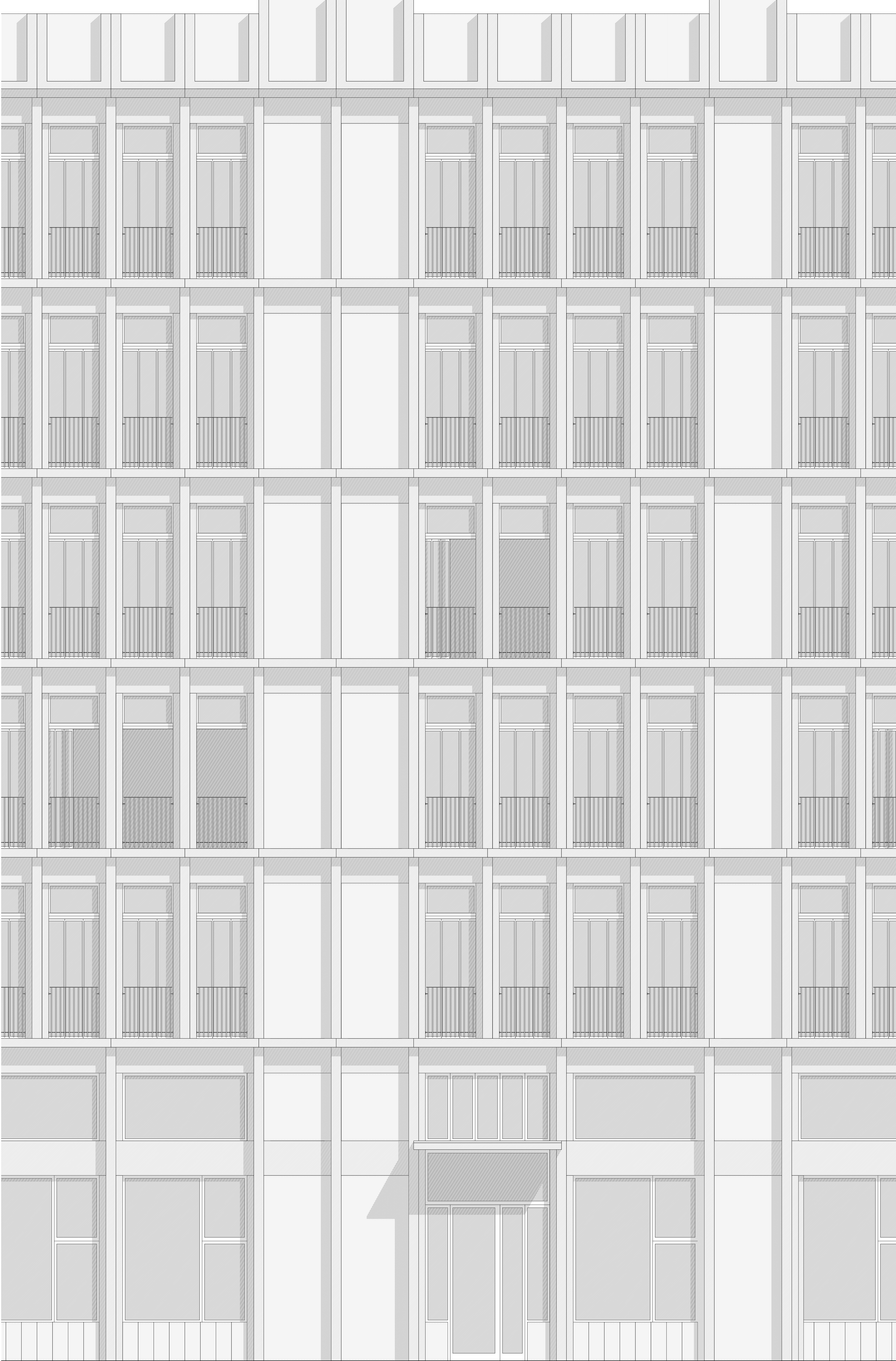
Fassadenausschnitt 1:33
