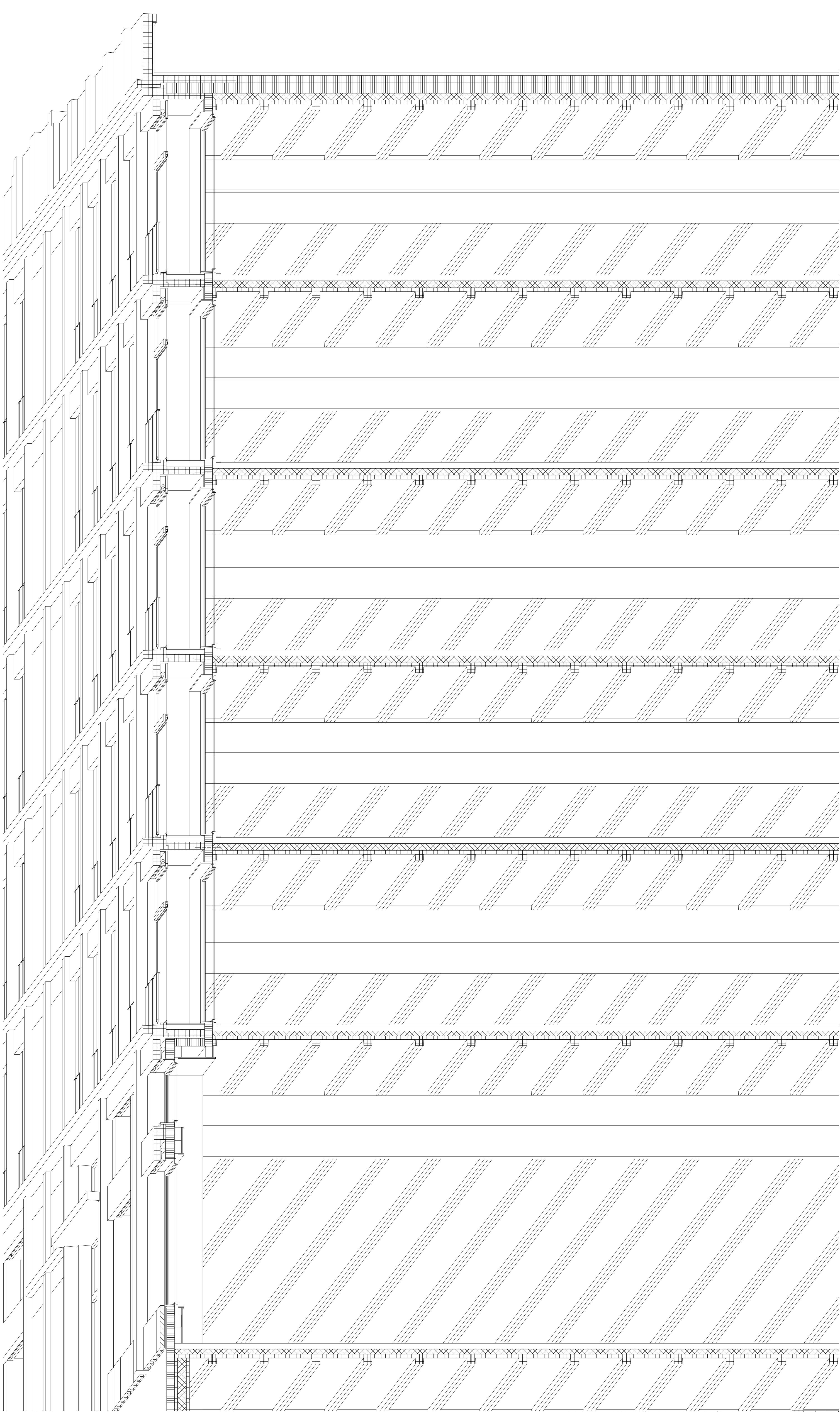
Fassadenschnitt 1:33
