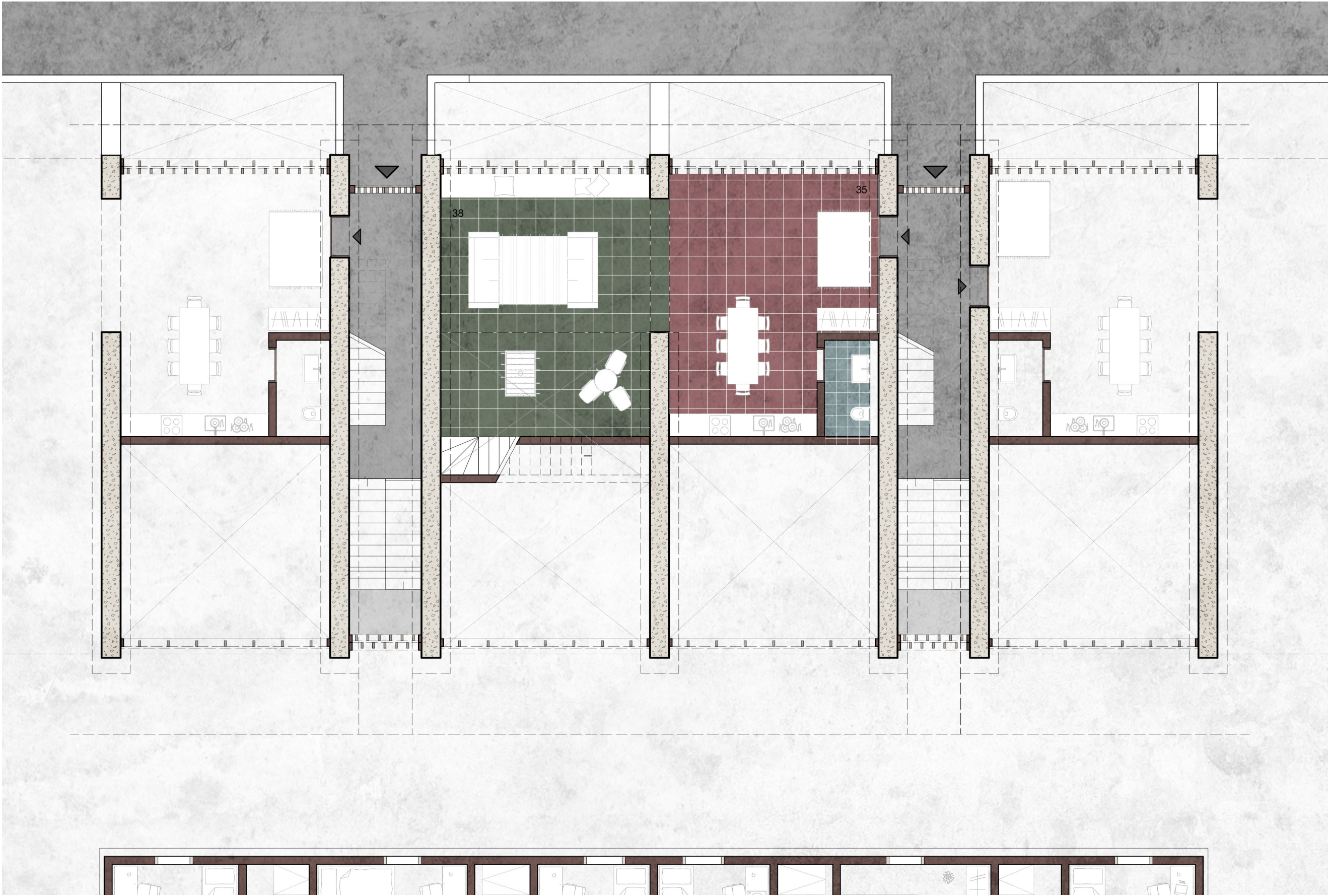
TYPOLGIE 3 - WOHNGESCHOSS WG | 1:100 |
