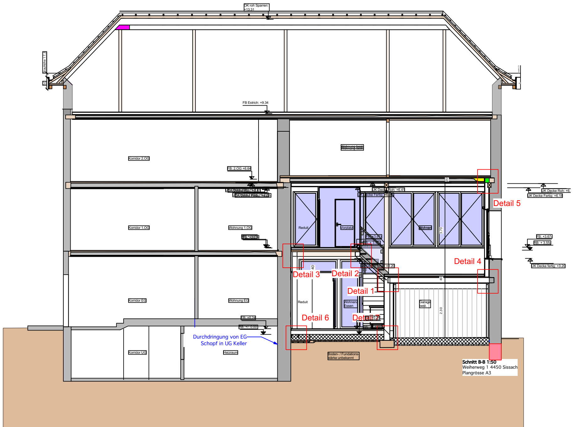
Schnitt B-B Masstab 1:100
