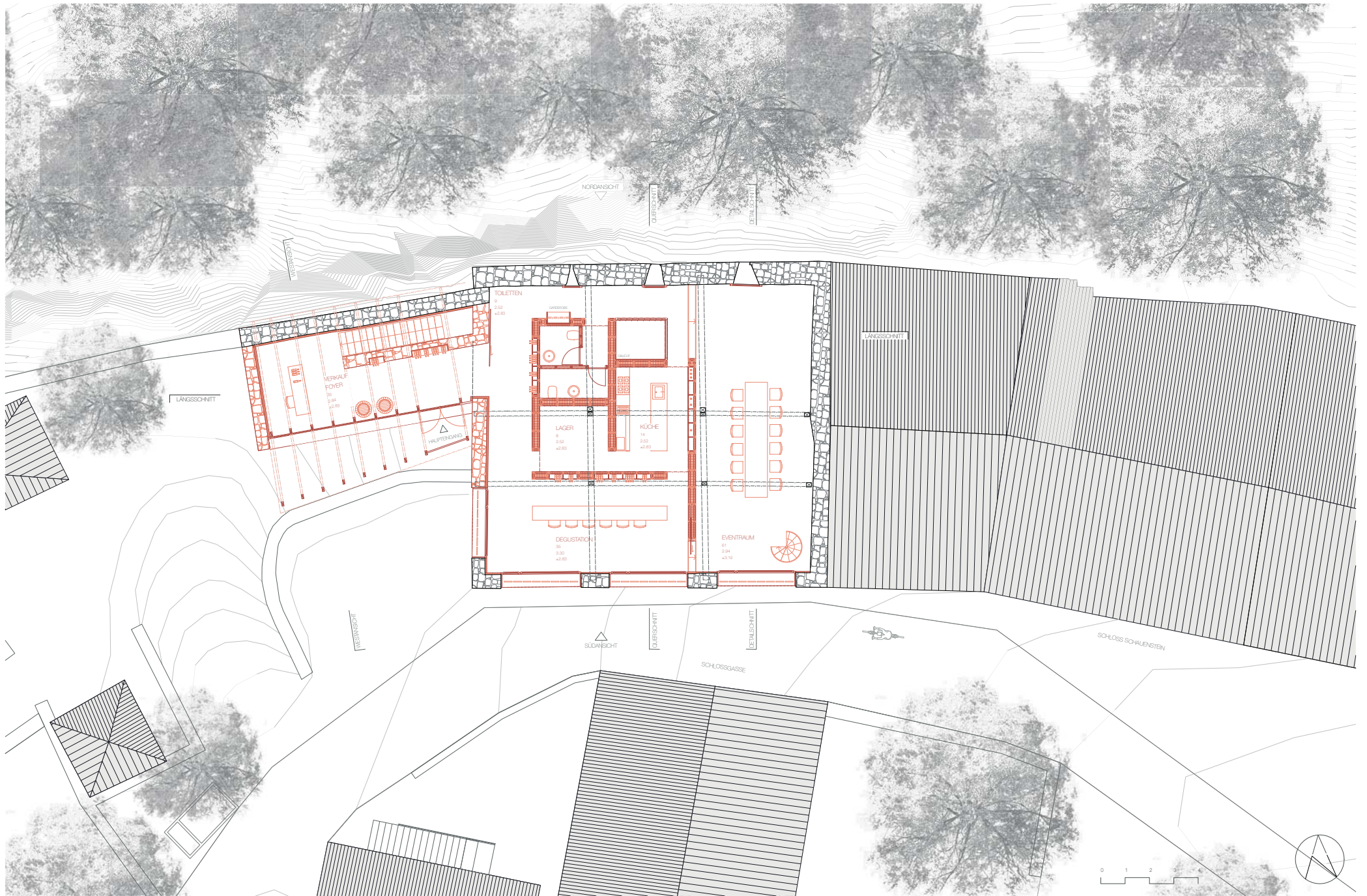
GRUNDRISS OBERGESCHOSS
