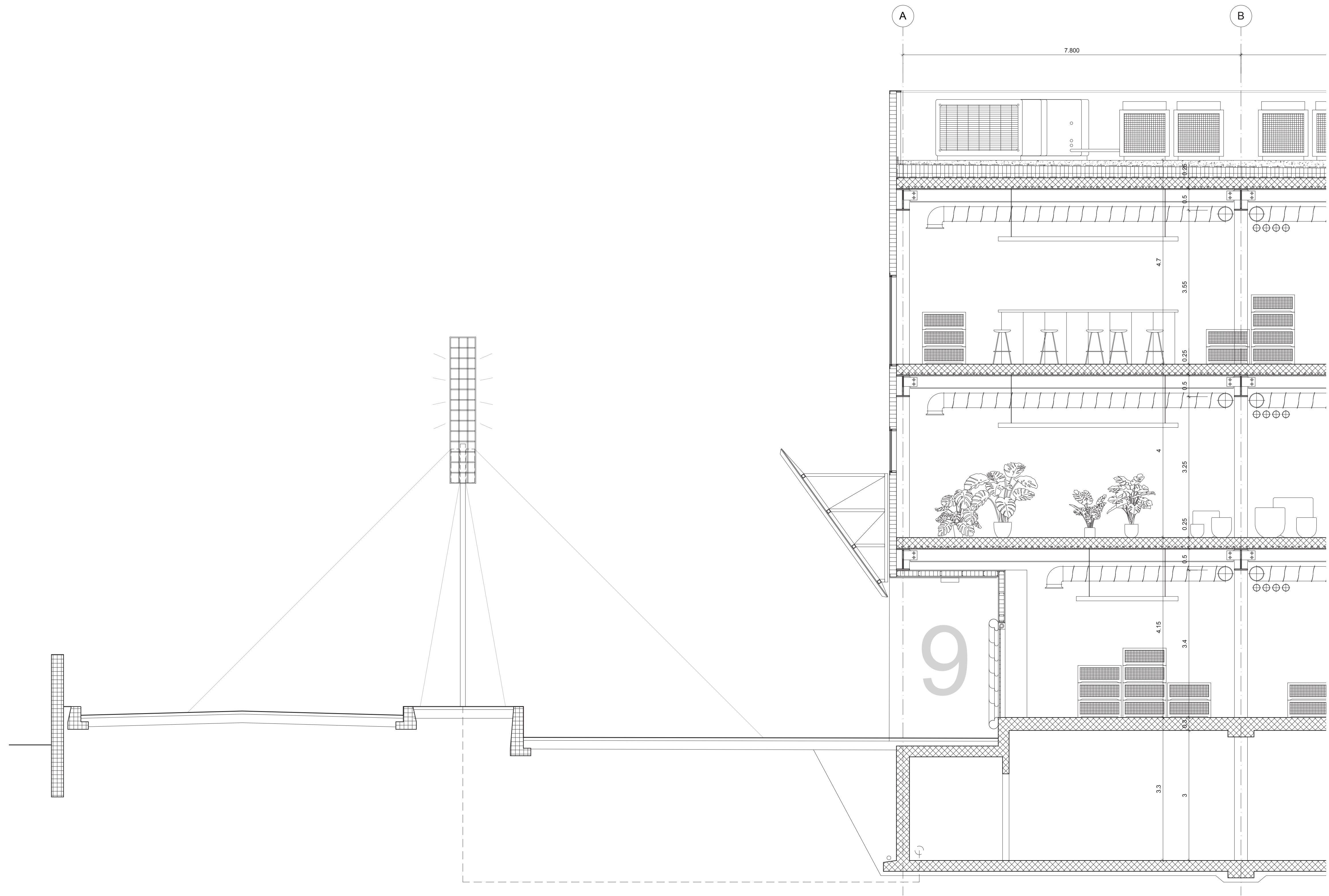
Coupe transversale - relation à la route Hub, 1:50
