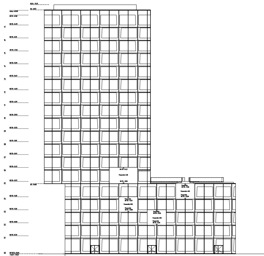
ALZADO 445
