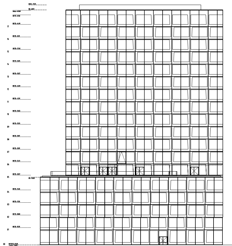
ALZADO 444
