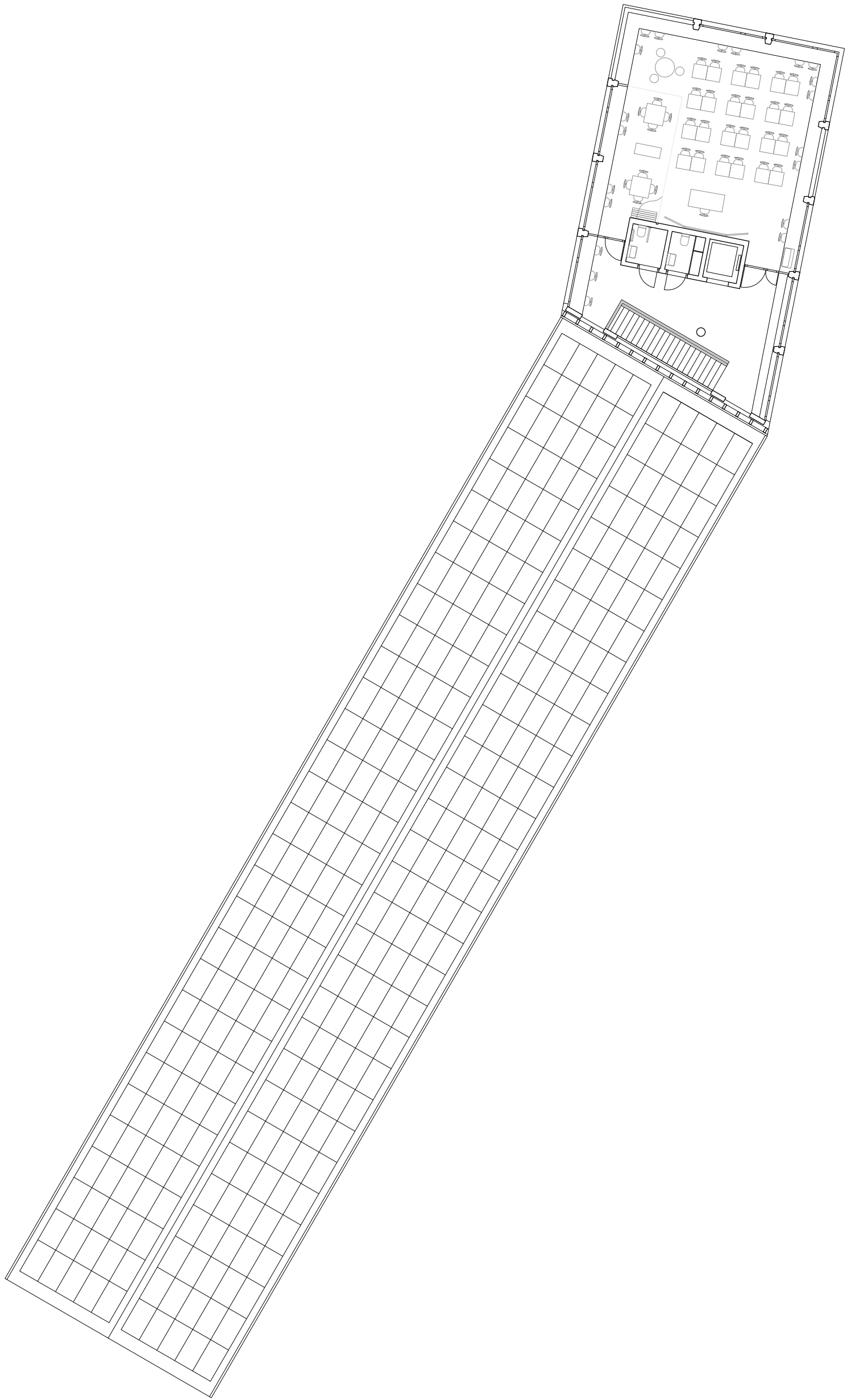
Obergeschoss 3 1:200
