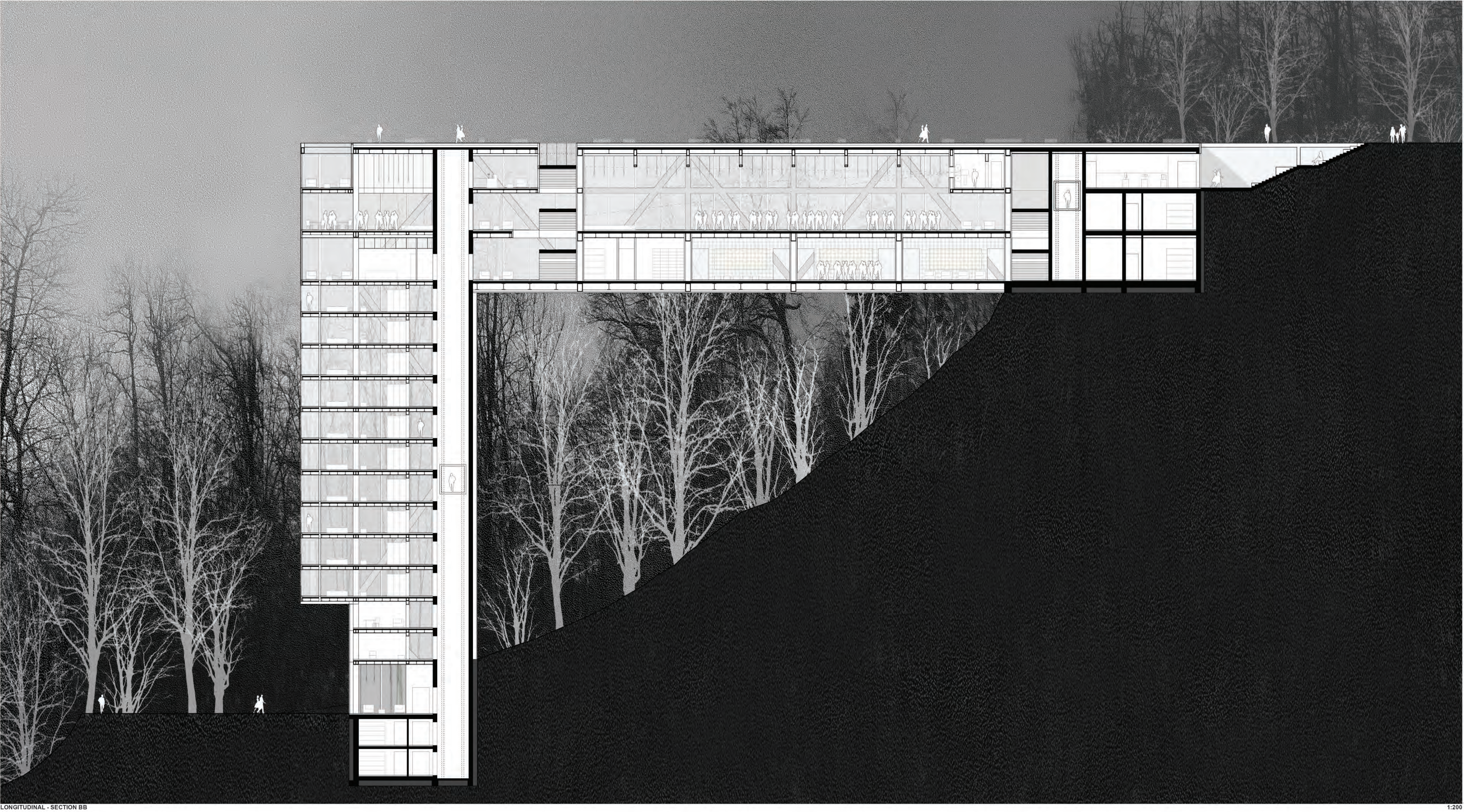
LONGITUDINAL - SECTION BB 1:200
