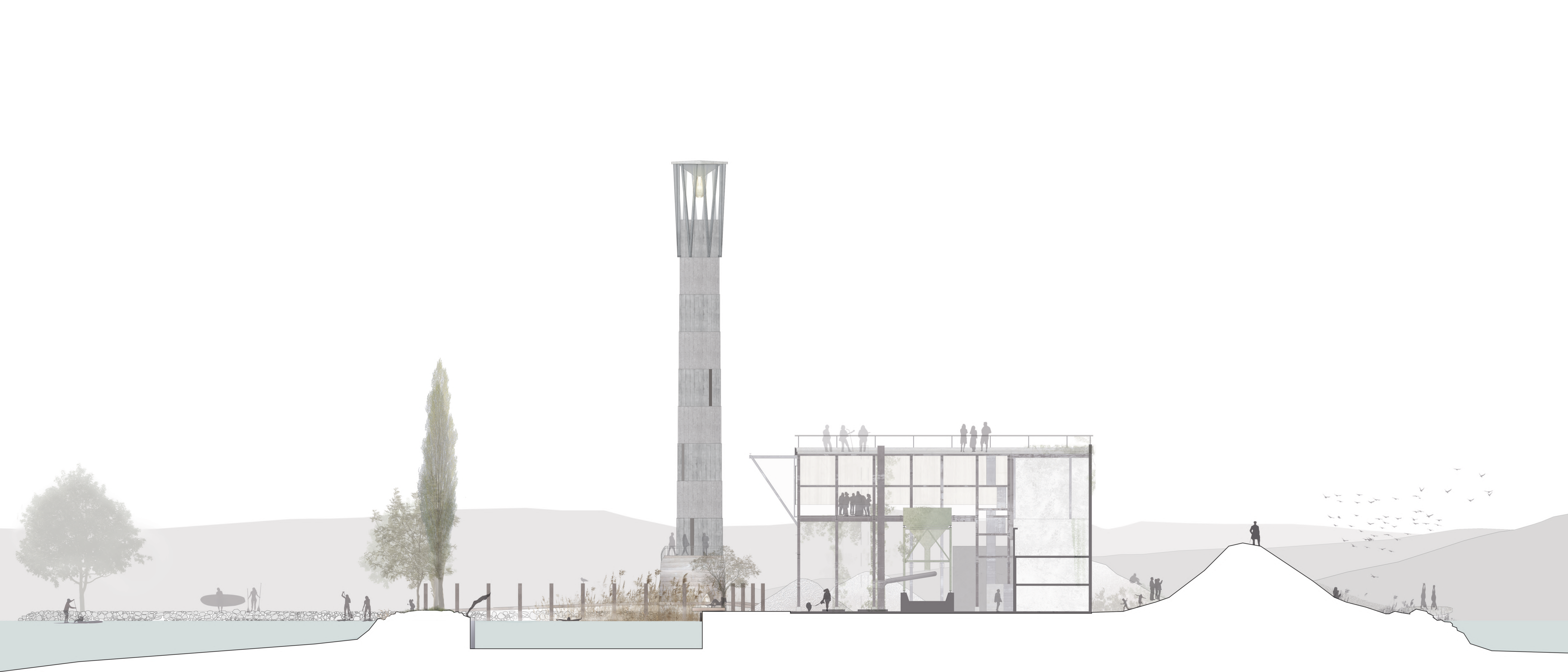
- COUPE STRUCTURE | 1:200 -
