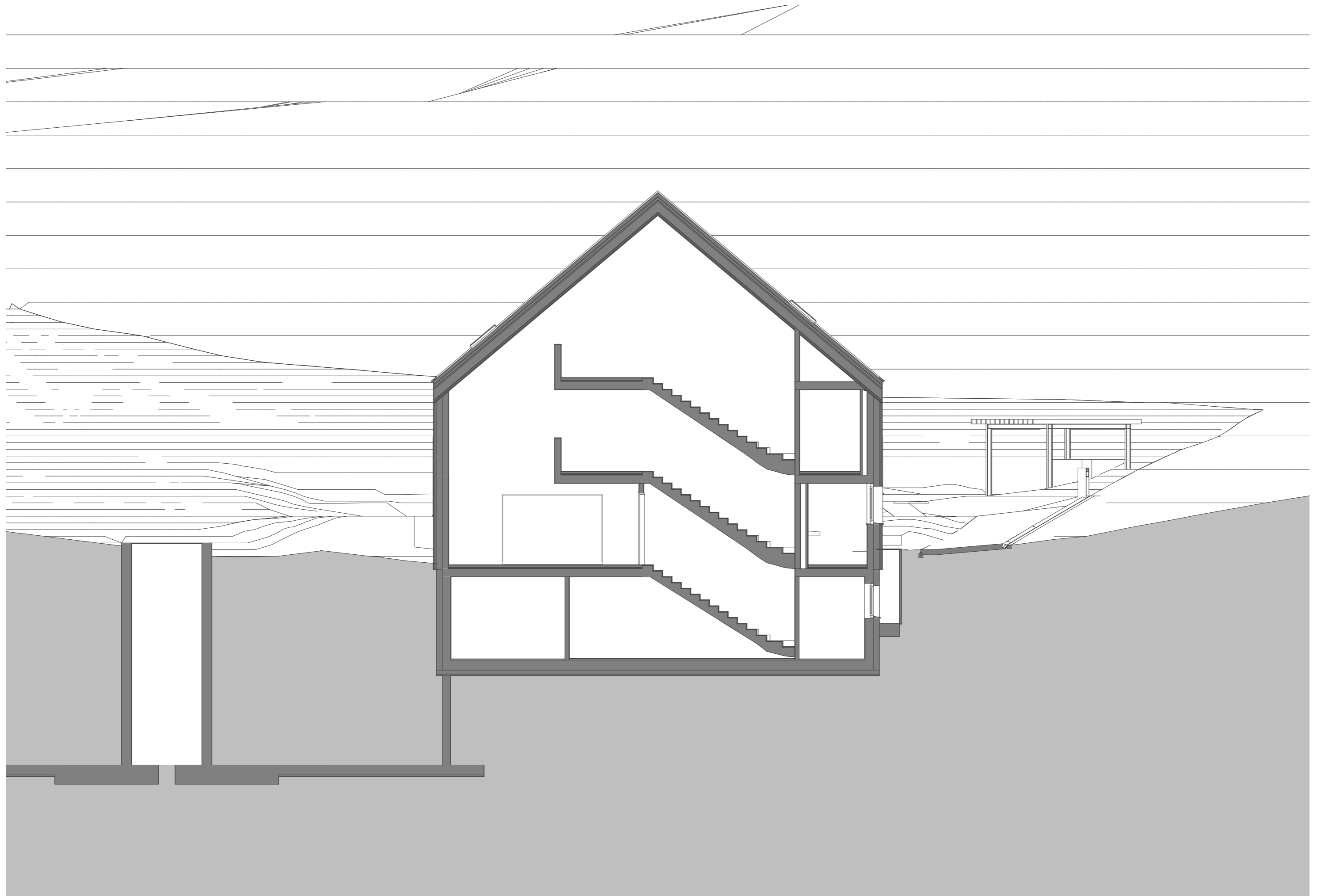
SCHNITT VI DEFH / 1:100
