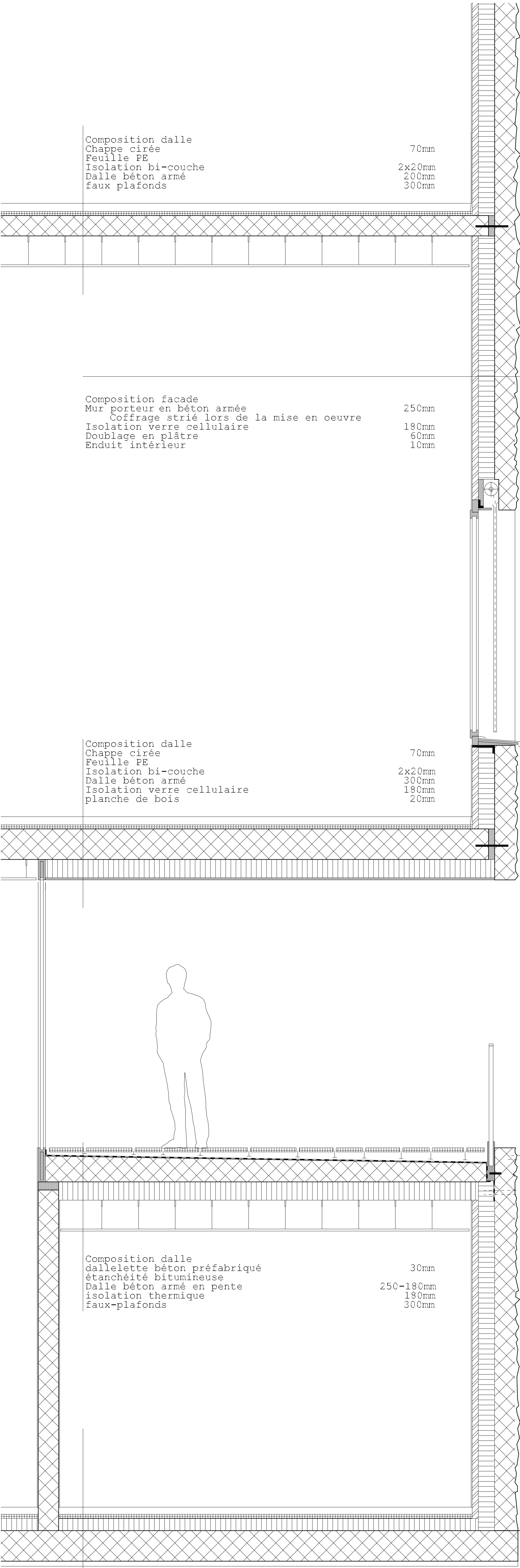
détail 1_20
