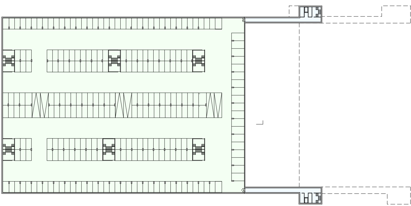
Grundriss -1.Untergeschoss 1_1000
