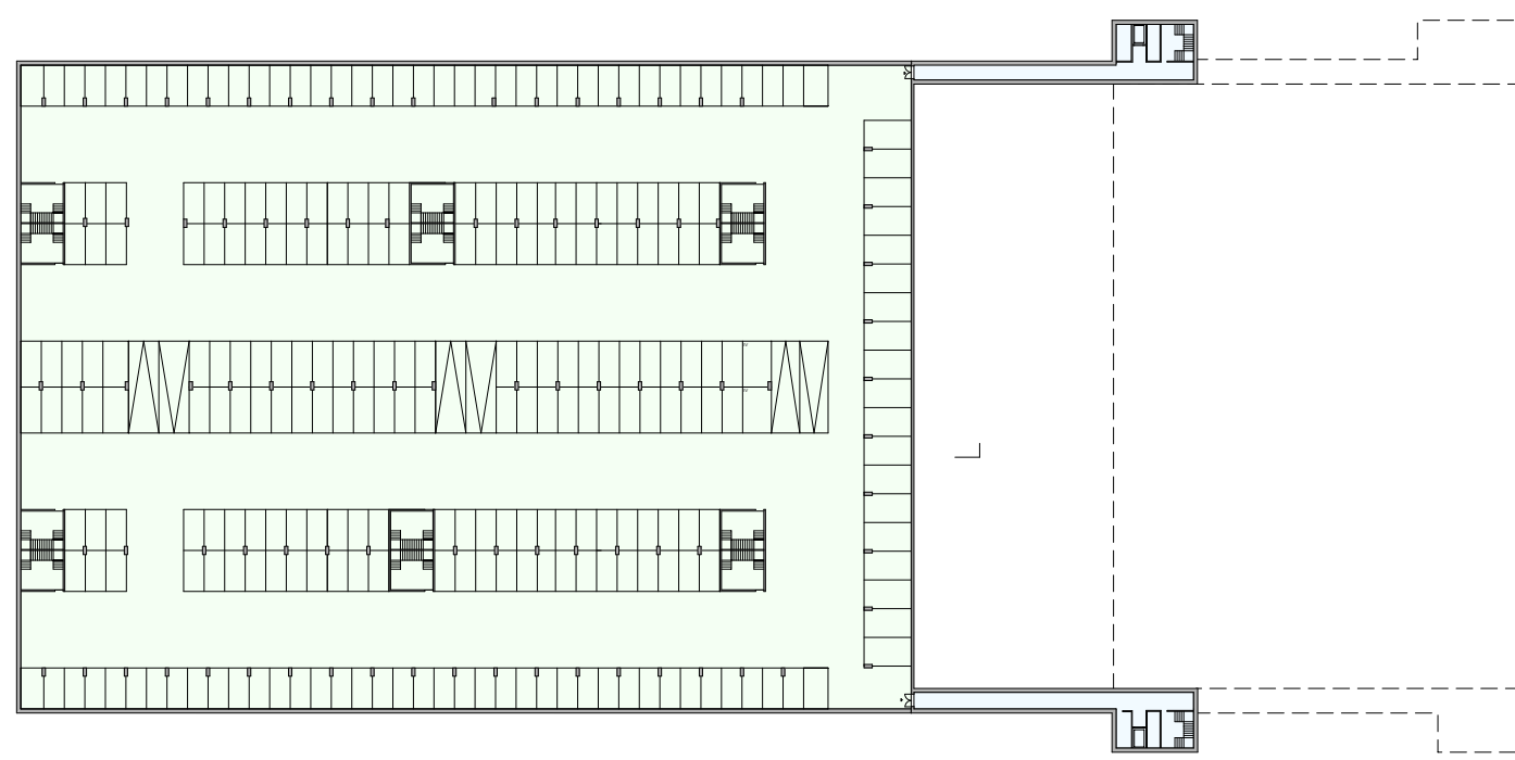
Grundriss -2.Untergeschoss 1_1000
