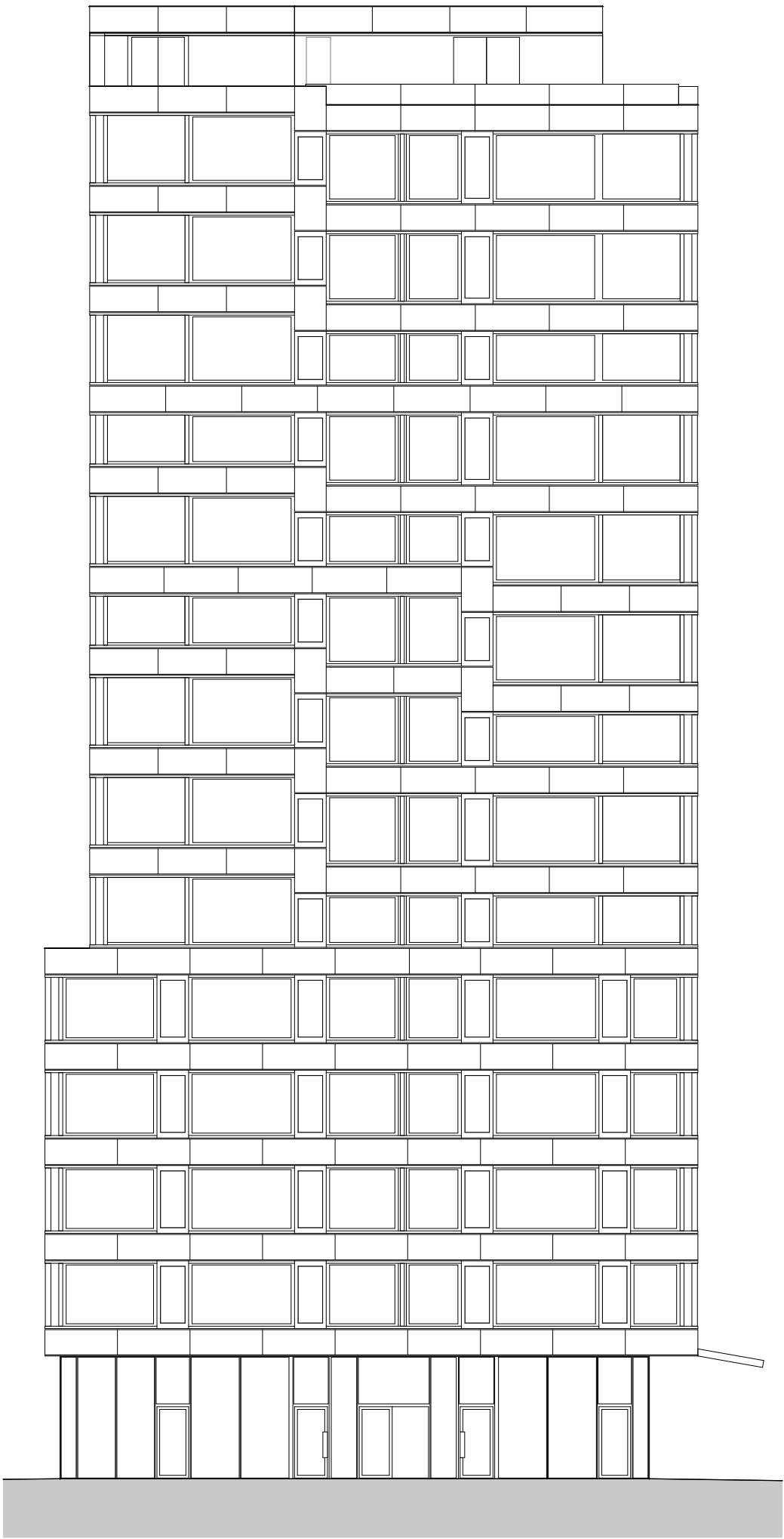
Ansicht WEST Zeichnungsmaßstab 1:200
