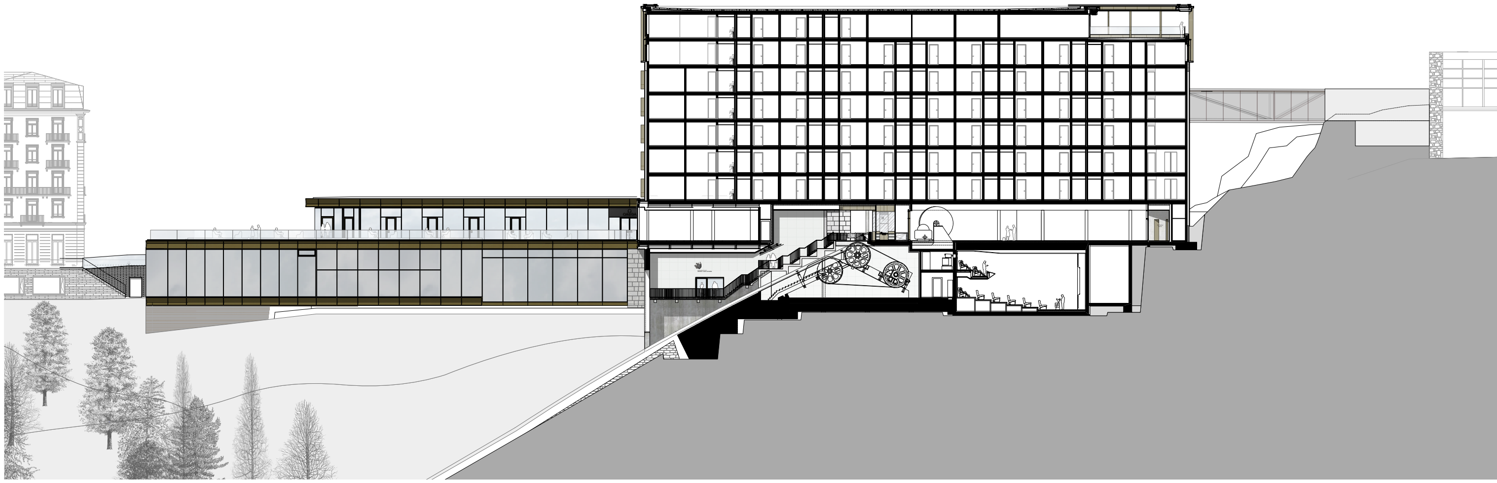
LÄNGSSCHNITT - BAHN & ZIMMERGESCHOSSE
