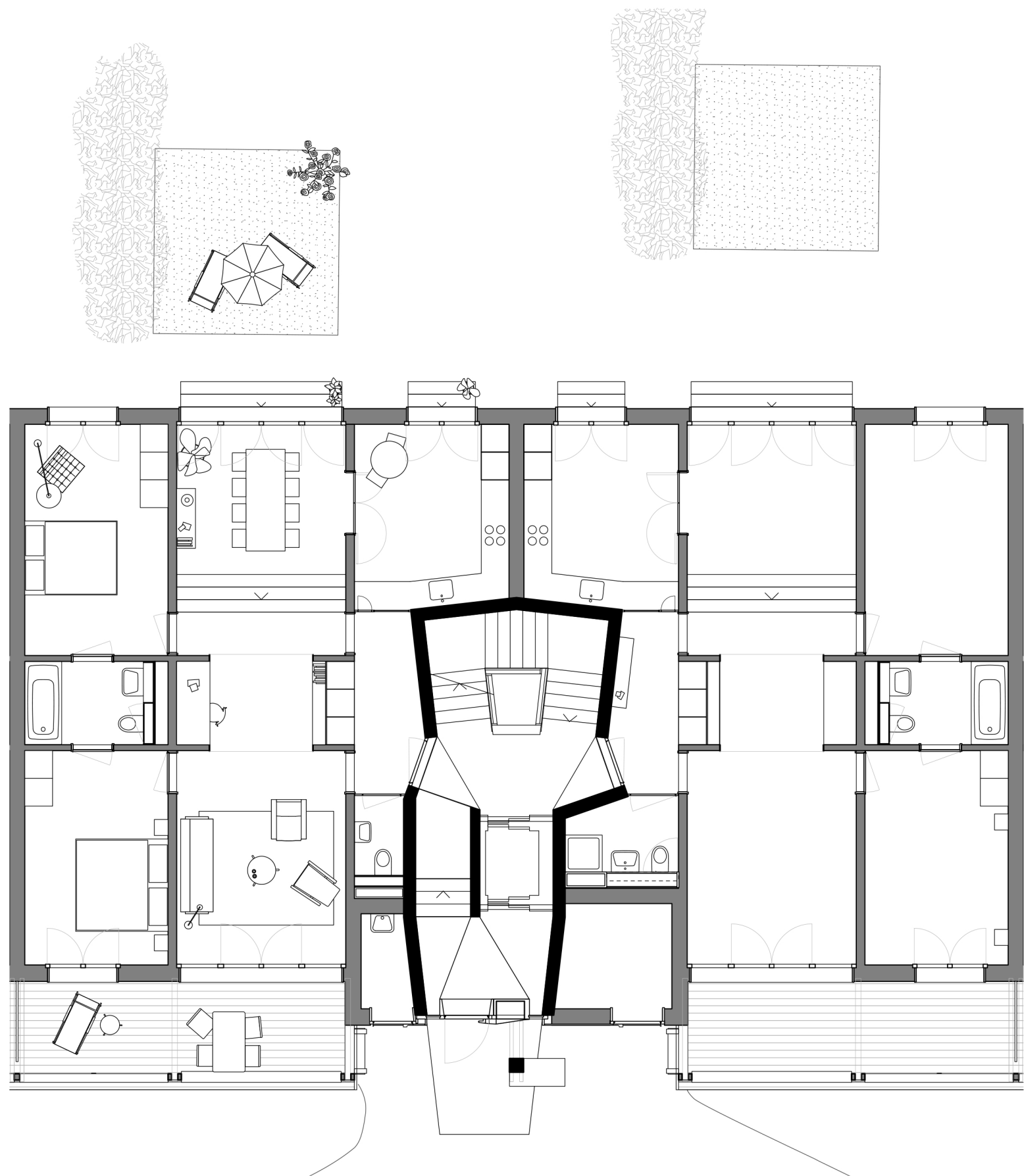
Wohnungstyp S-Haus EG
