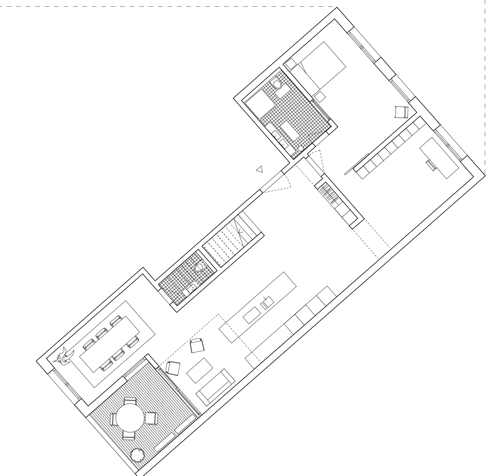
Wohnung Maisonette 1:100 6.5 Zimmer 190 m 2
