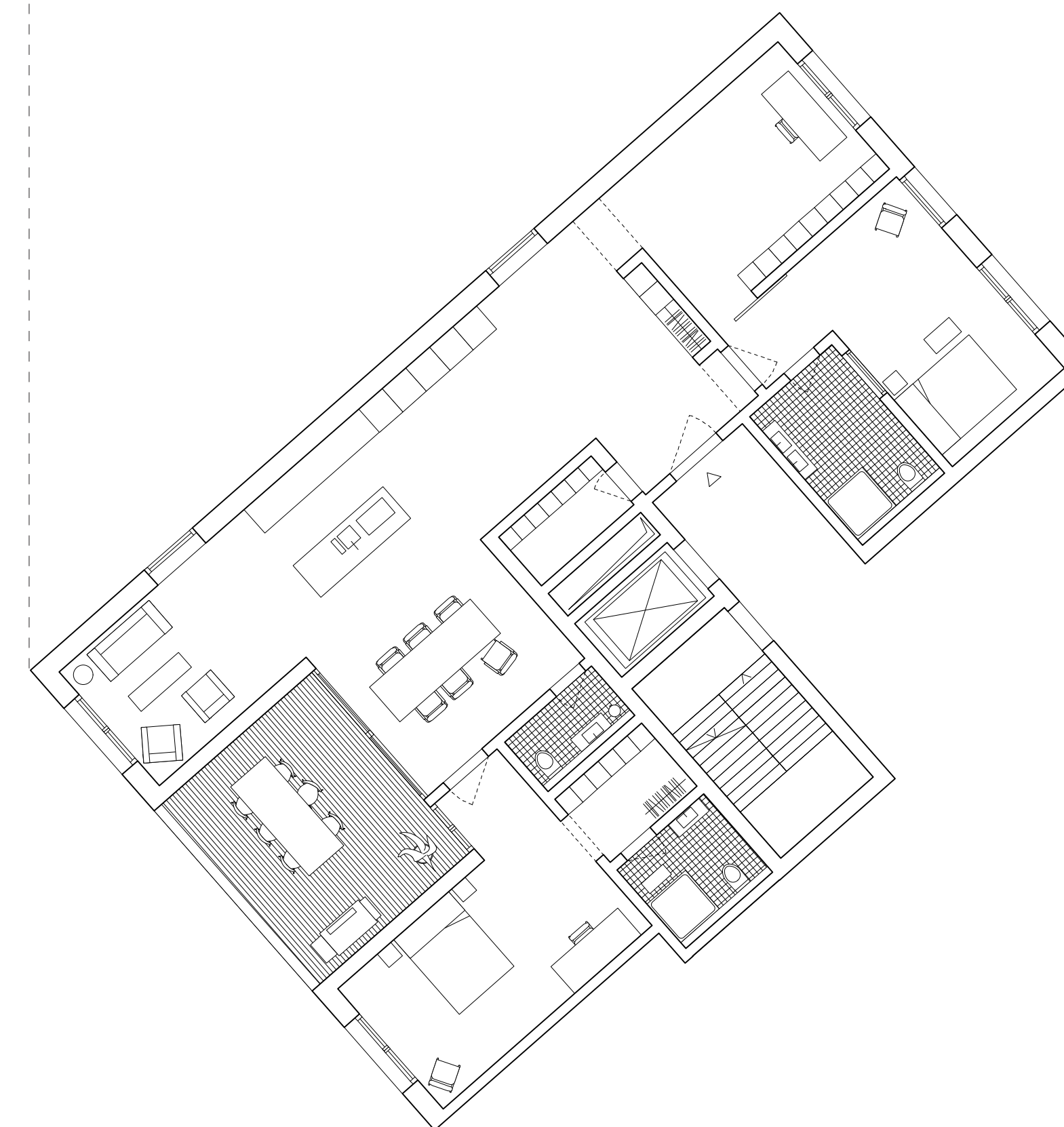
Wohnung I 1:100 4.5 Zimmer 154 m 2
