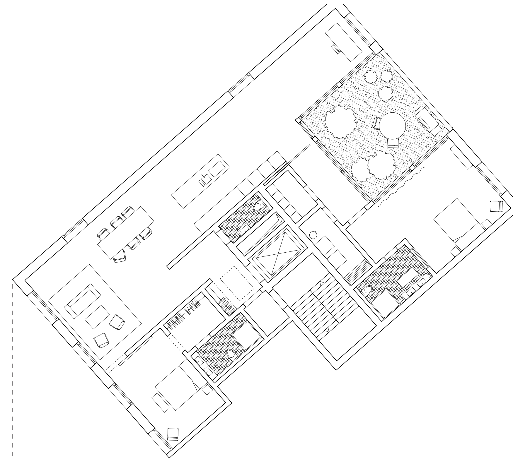
Wohnung II 1:100 4.5 Zimmer 157 m 2
