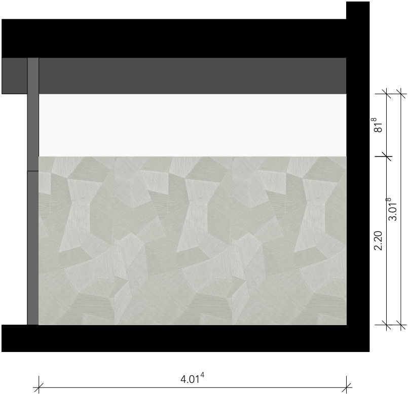
SCHNITT F-F
