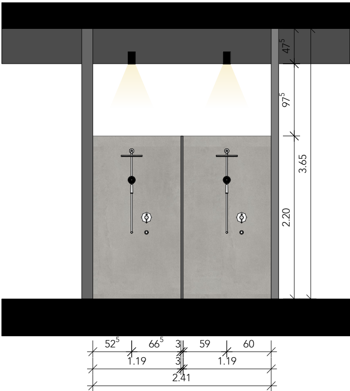
SCHNITT L-L
