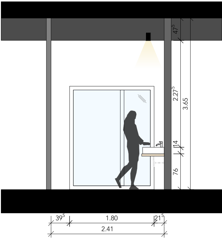
SCHNITT M-M
