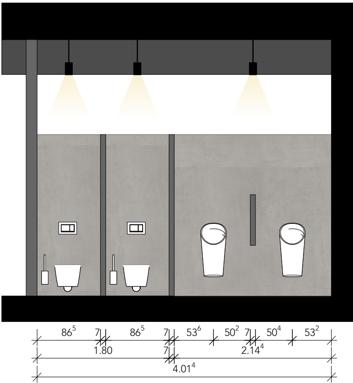
SCHNITT H-H
