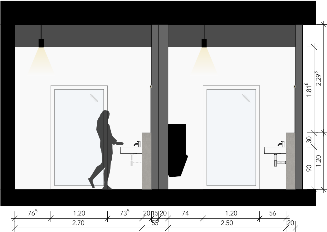
SCHNITT H-H
