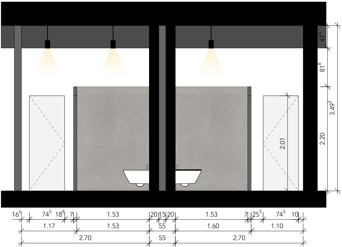
SCHNITT M-M
