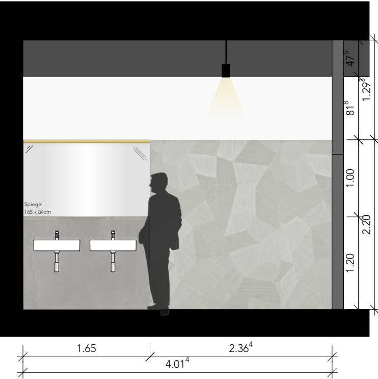
SCHNITT G-G
