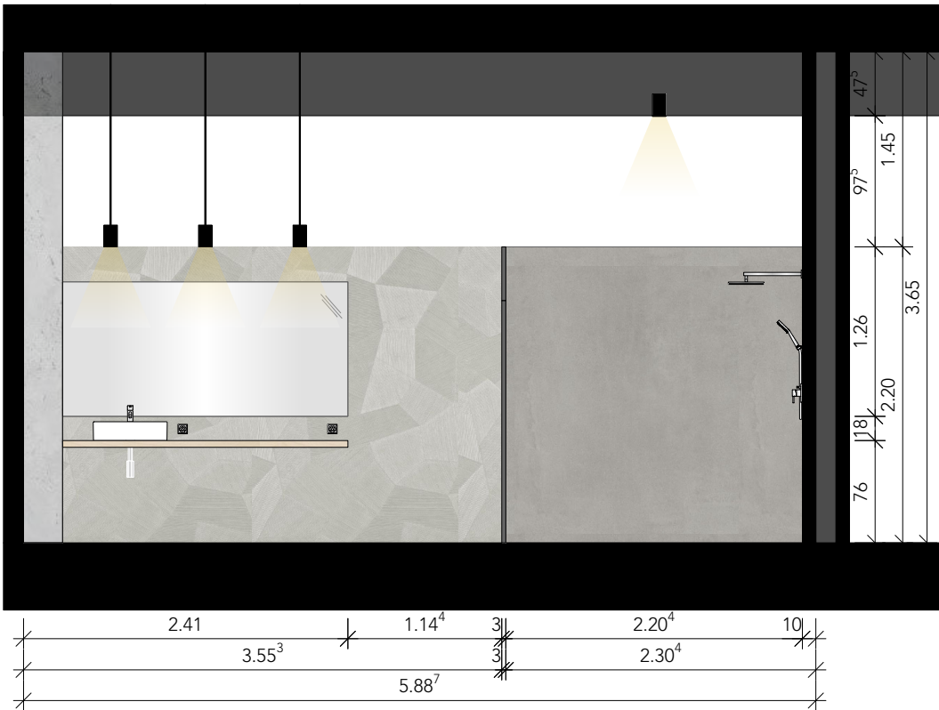
SCHNITT K-K
