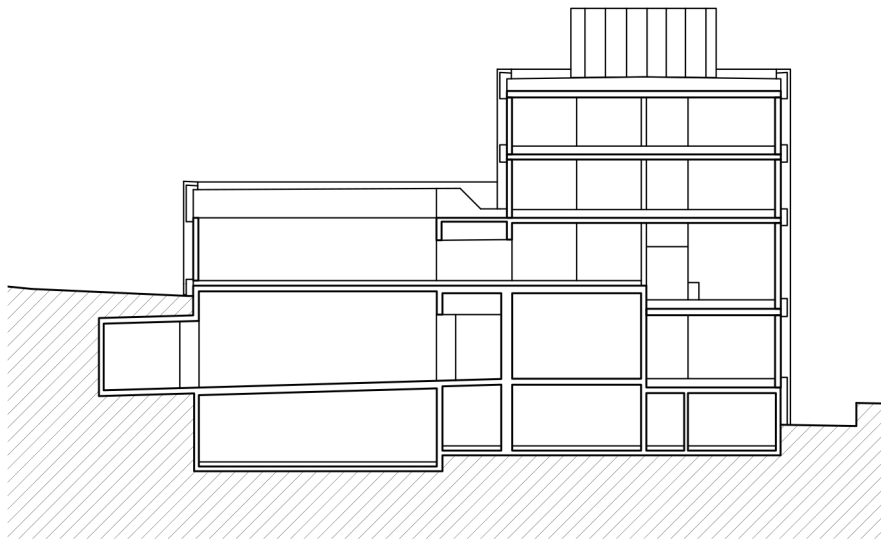
Coupe transversale
