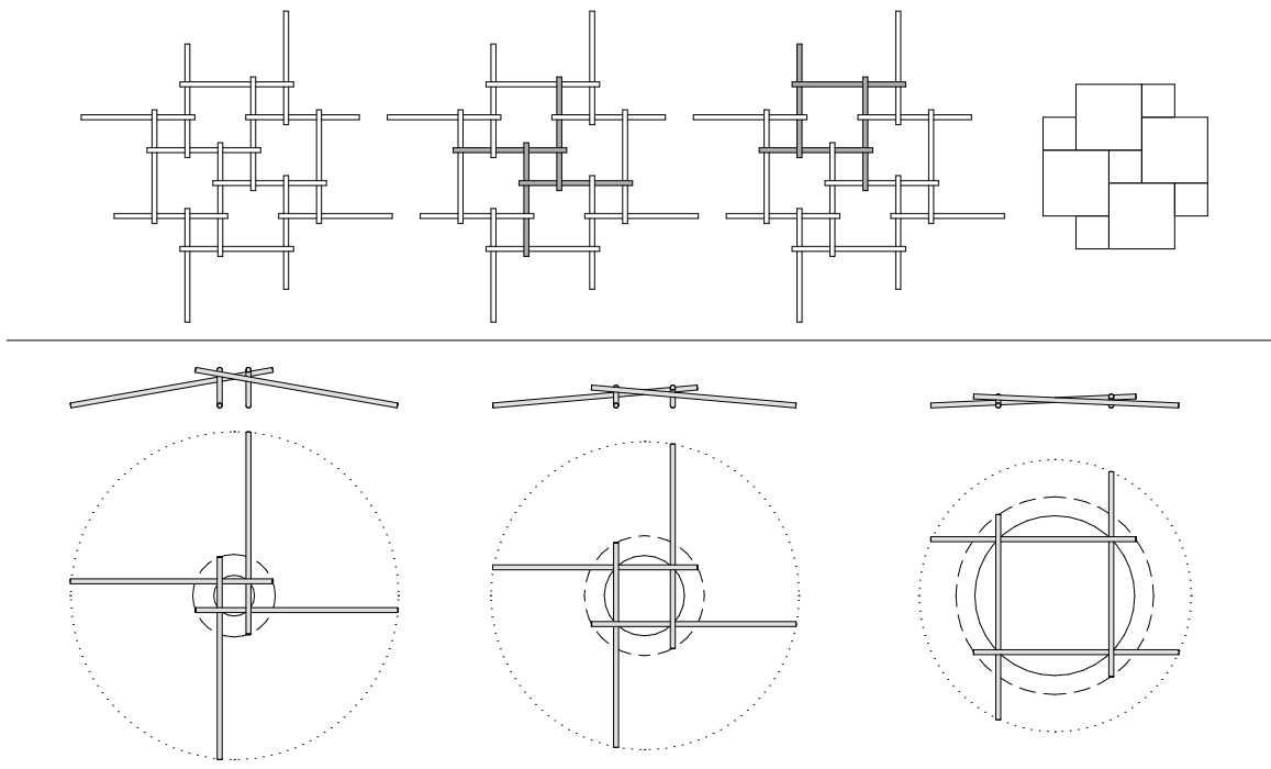
Hebelstabwerk
