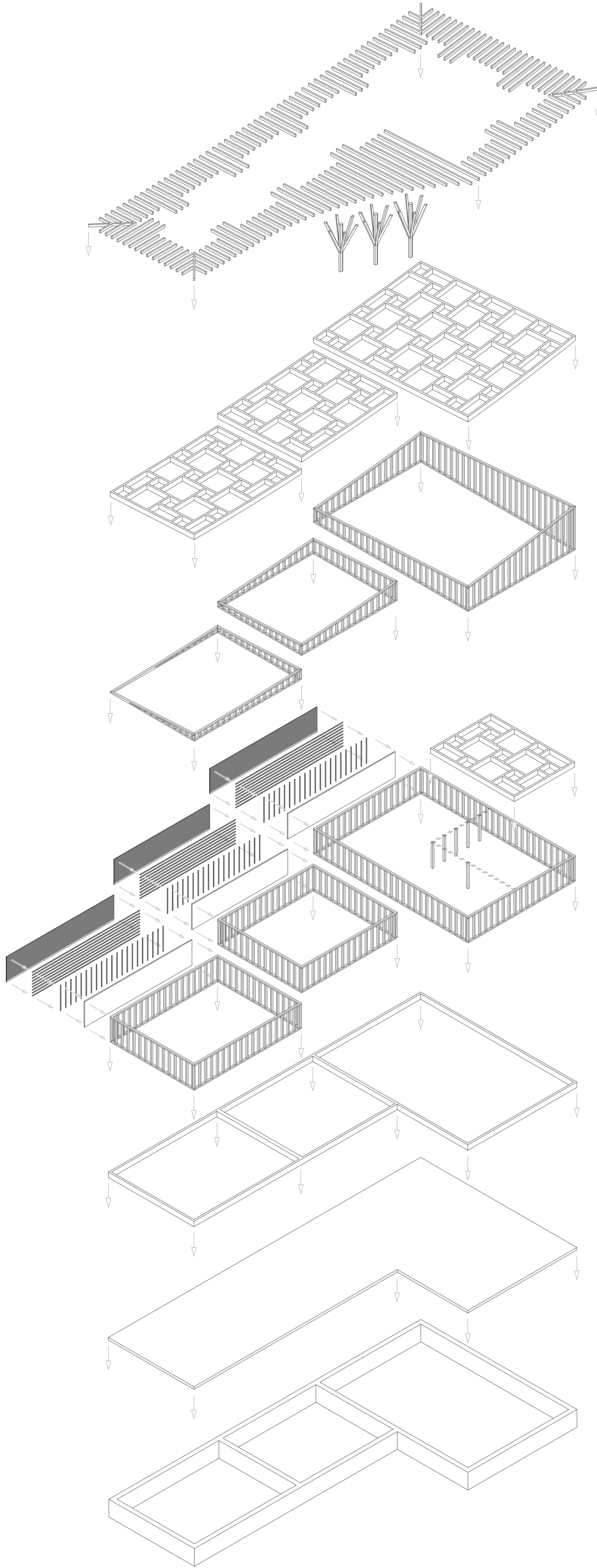
Explosionszeichnung Bauablauf | 200
