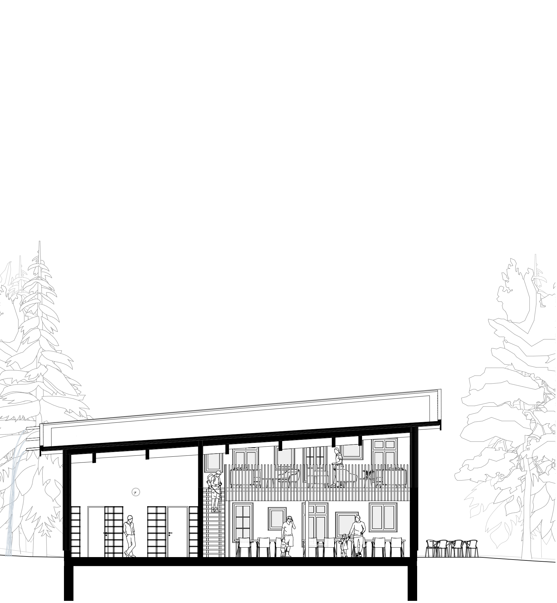
Schnitt | 100
