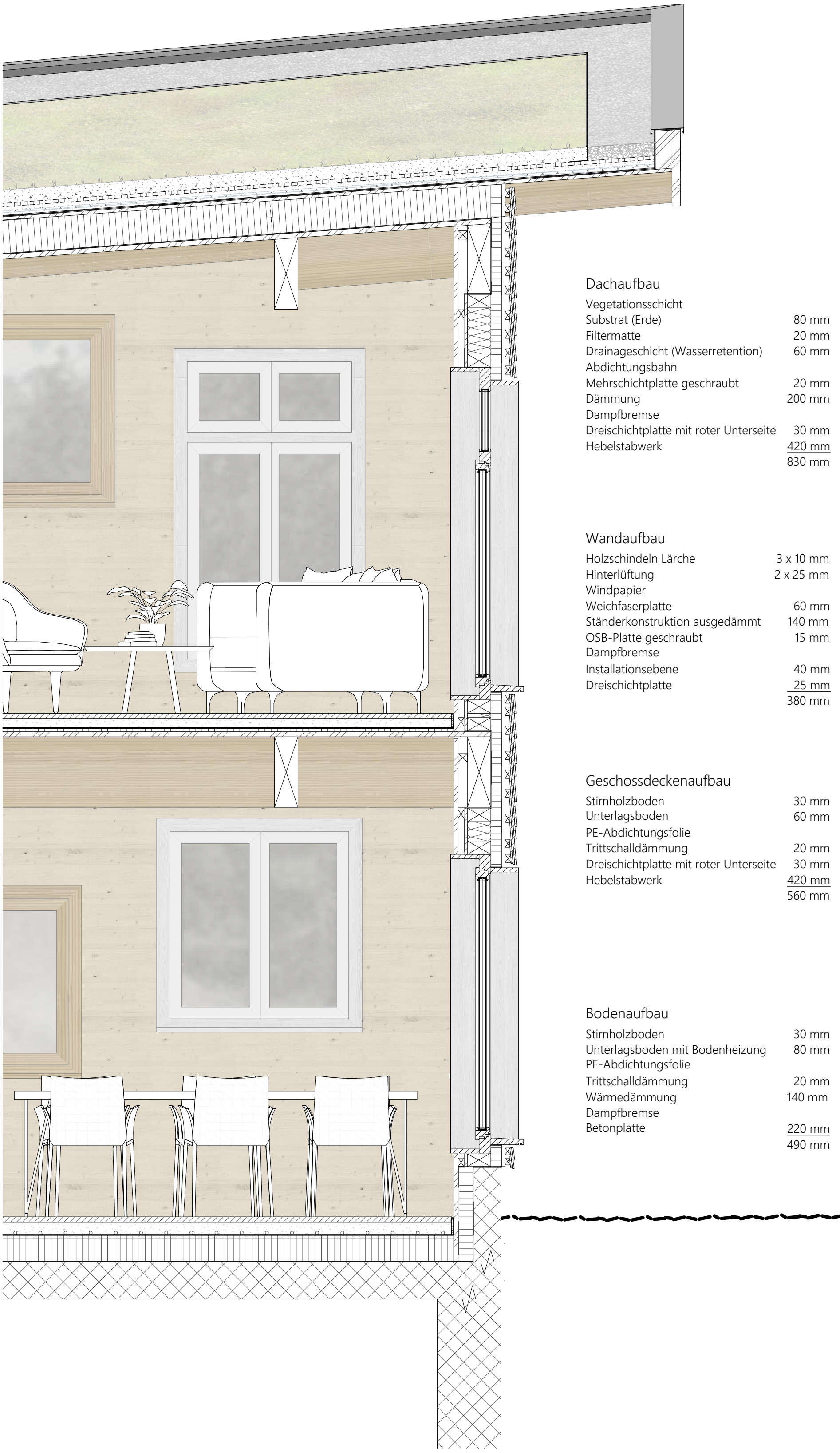
Konstruktionsschnitt | 20
