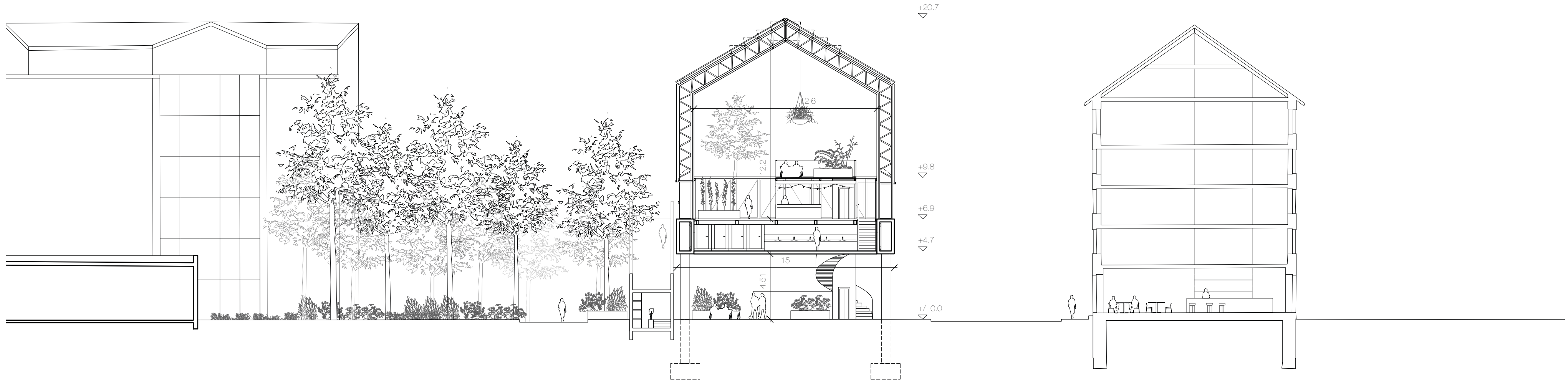
1:200 Schnitt 3-3
