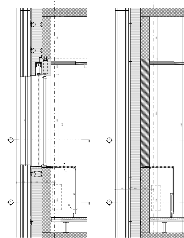
Typische Wandschnitte
