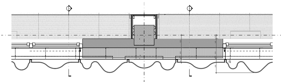
Planausschnitt durch Fenster
