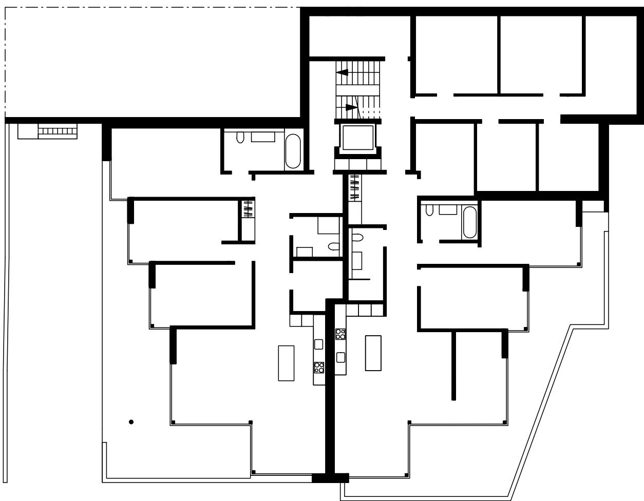
SOCKELGESCHOSS
