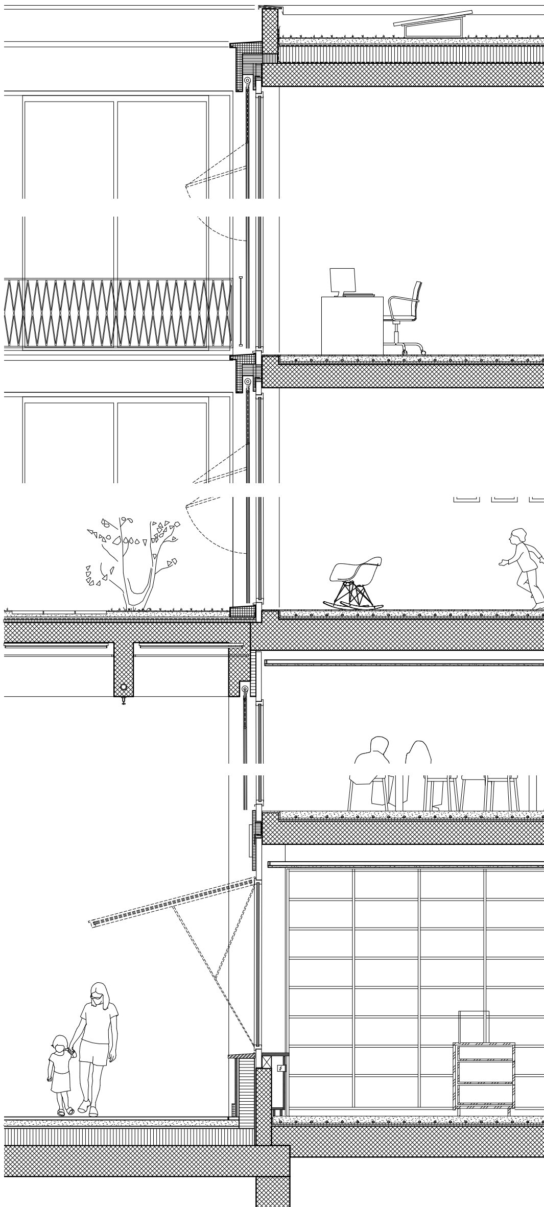
Konstruktionsdetails 1:50
