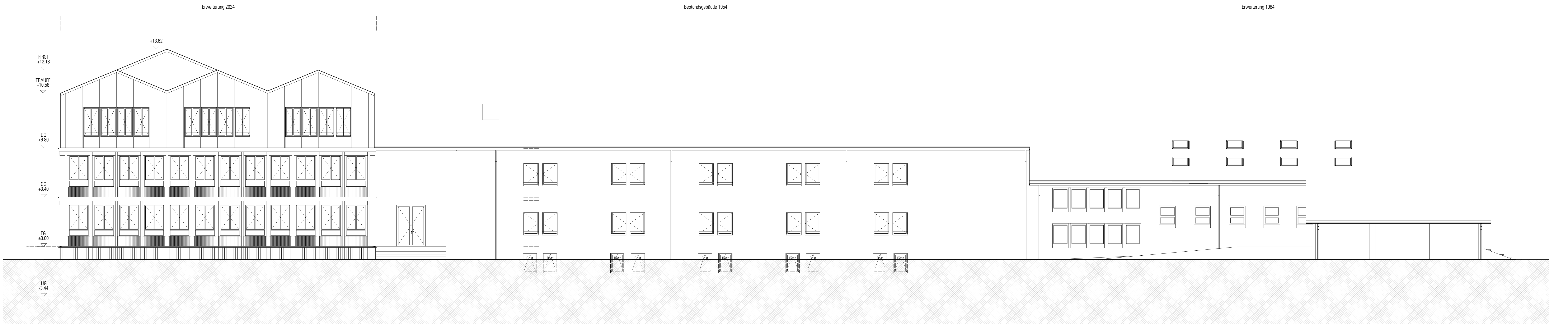
Fassade Nordwest
