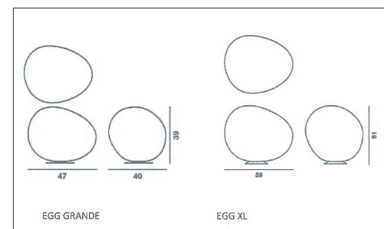
DETTAGLIO 3 Lampade da giardino EGG Max XL dim. 59x51x49 EGG Grande dim. 47x40x39
