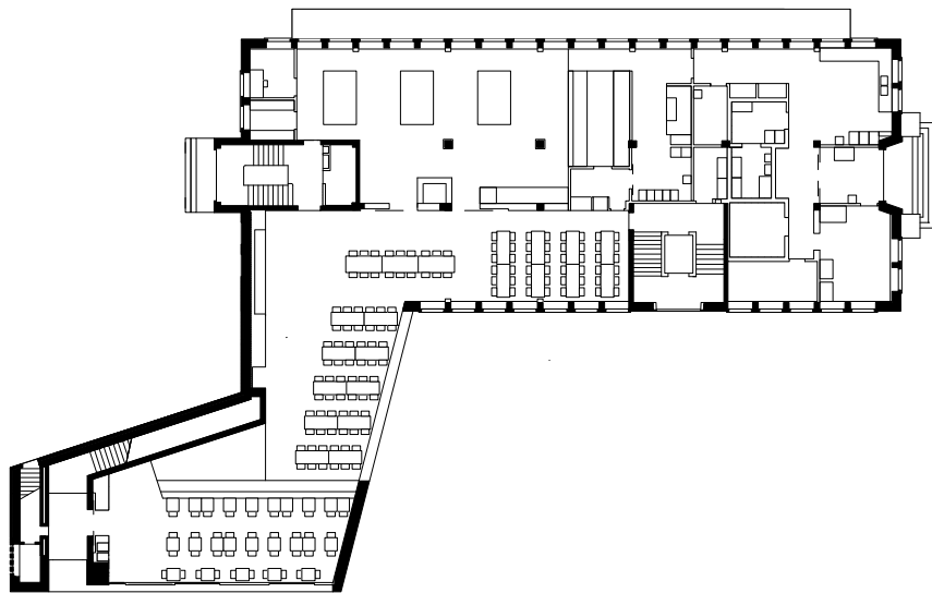
Erdgeschoss 1:500
