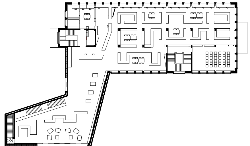
1. Obergeschoss 1:500
