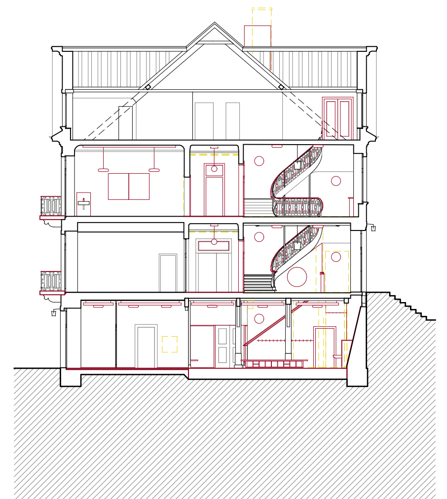
Querschnitt
