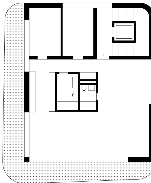
Grundriss 2. OG
