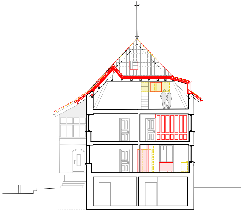
Längsschnitt
