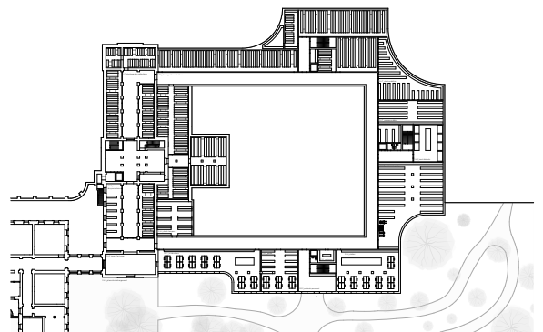
rez-inférieur 1_500
