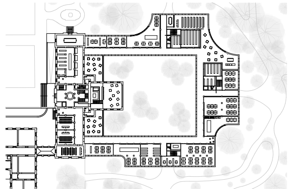
rez-supérieur 1_500
