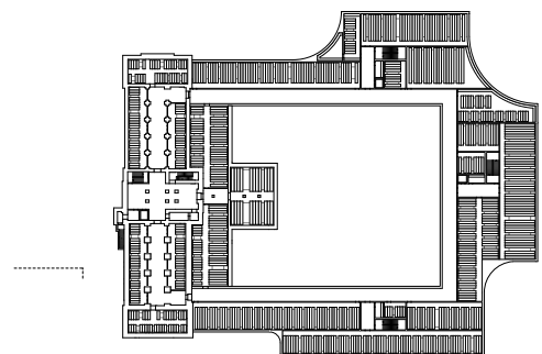
sous-sol -1, -2 1_500
