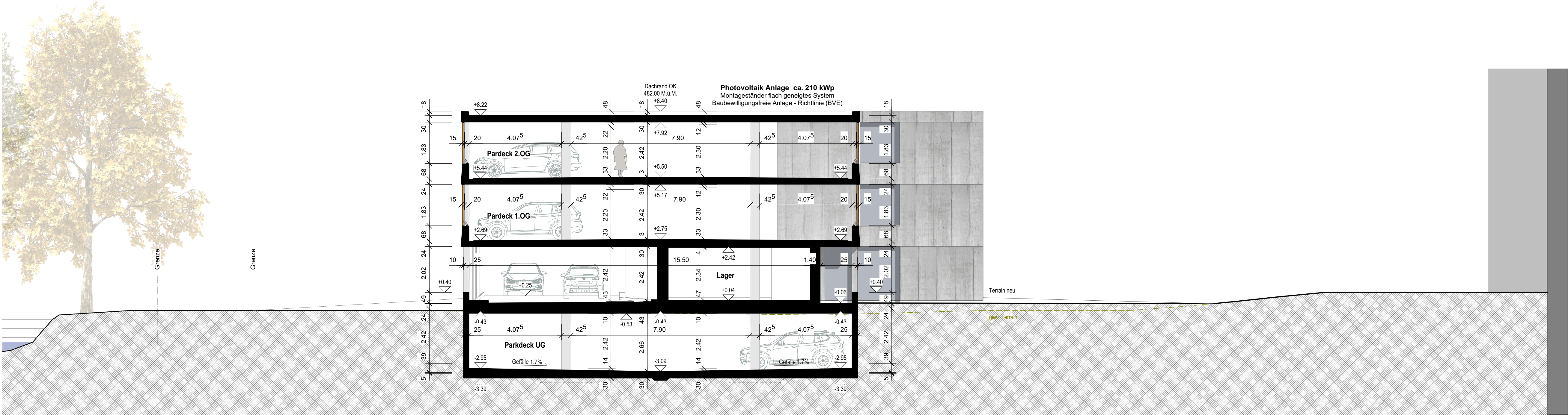
Schnitt E-E
