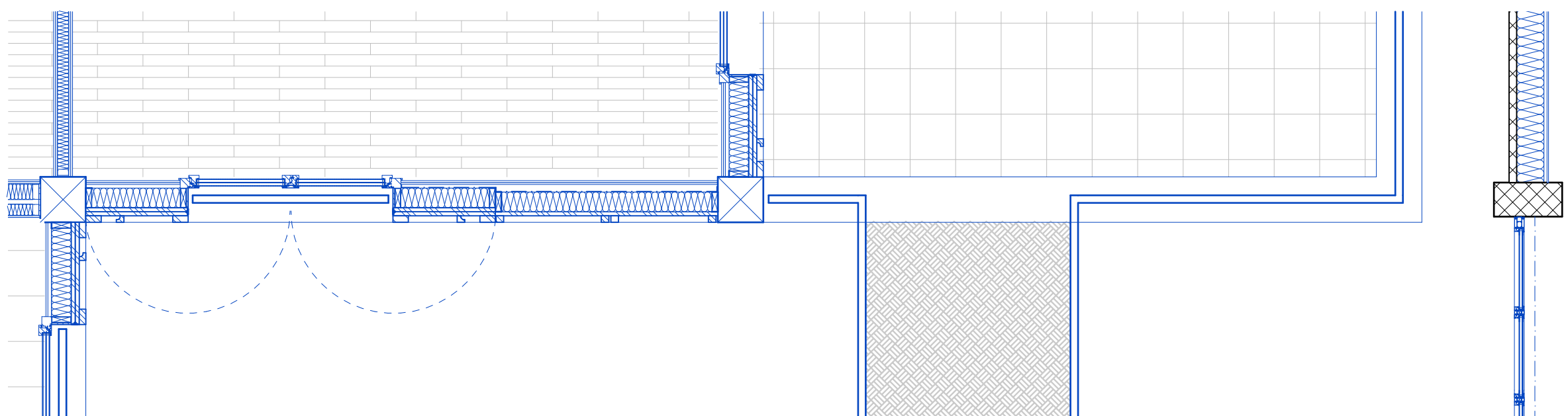
Detailgrundriss 1.Obergeschoss | 1:33
