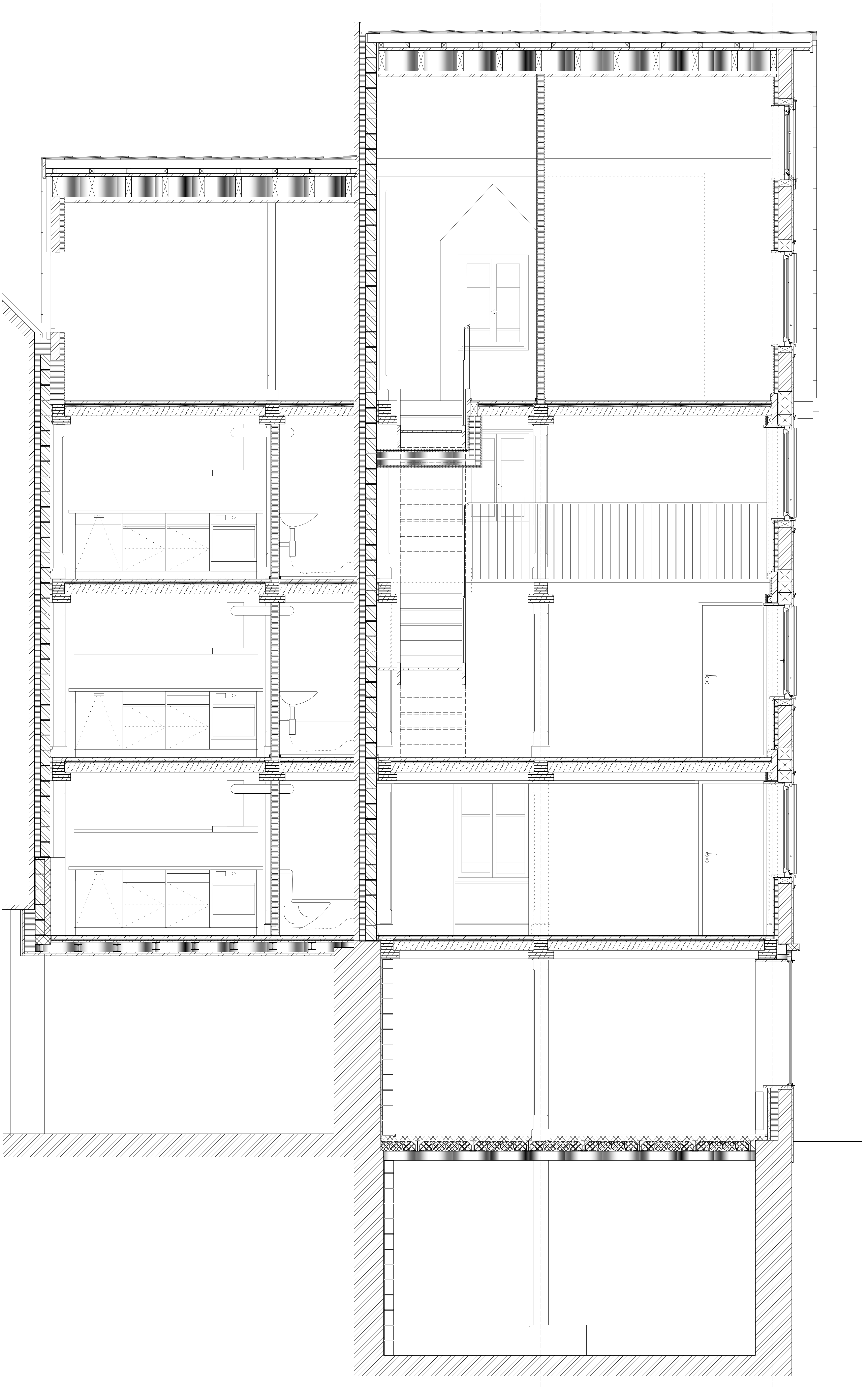
Querschnitt
