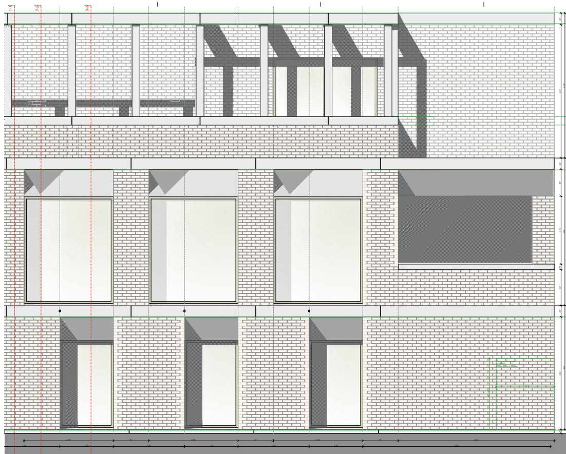
Teilansicht Fassade Süd
