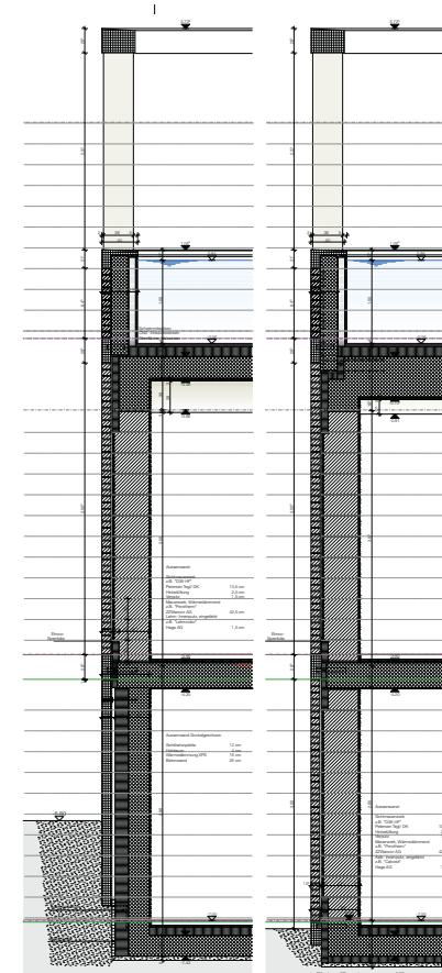
Vertikalschnitt Fassade West
