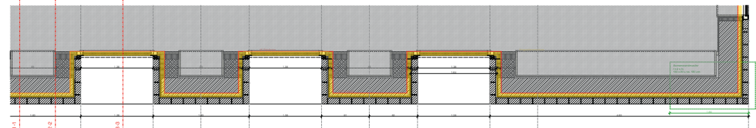
Horizontalschnitt Fassade Süd Ebene 02
