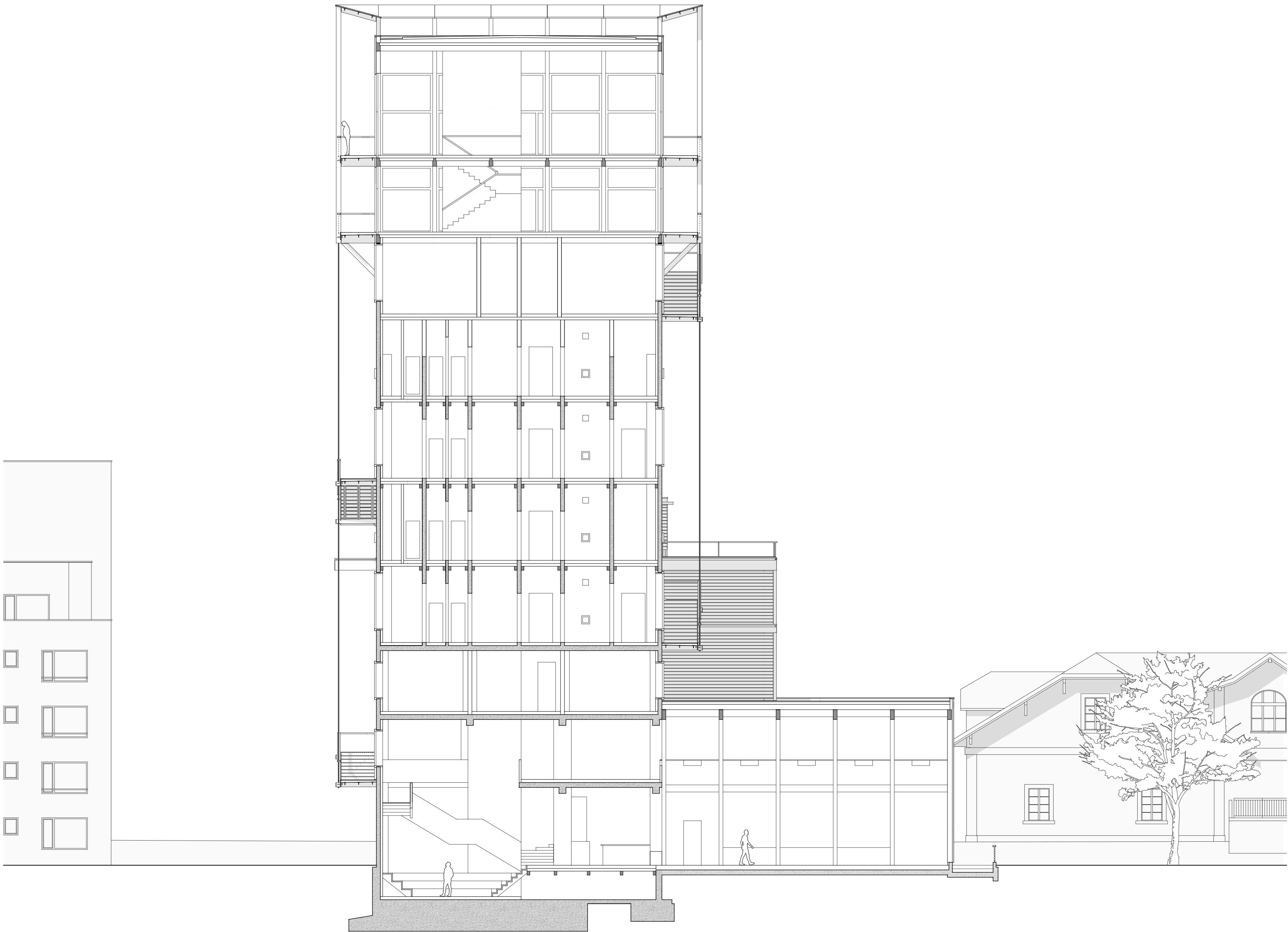
Querschnitt Nord 1_150
