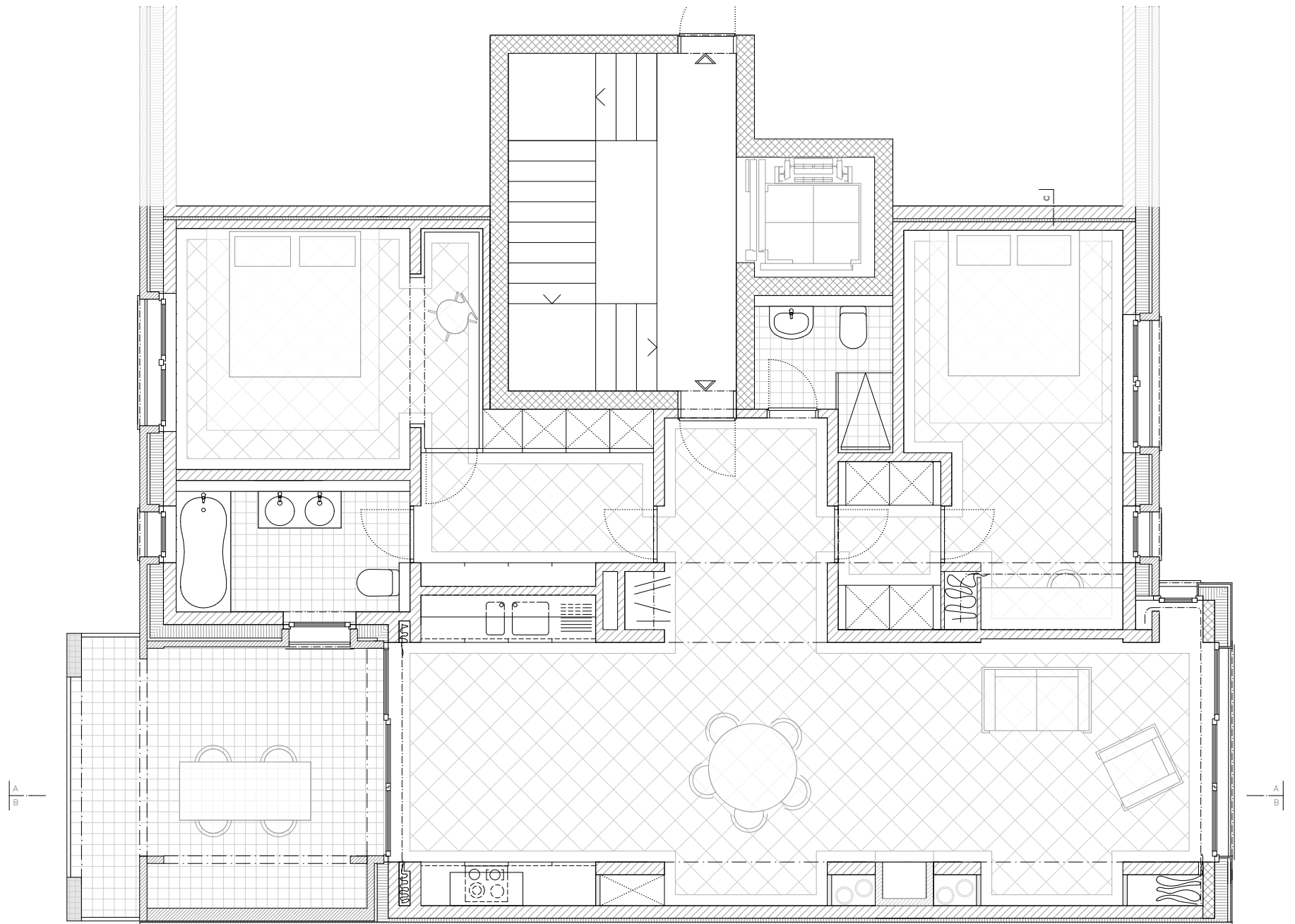
Grundriss Wohnung Level up
