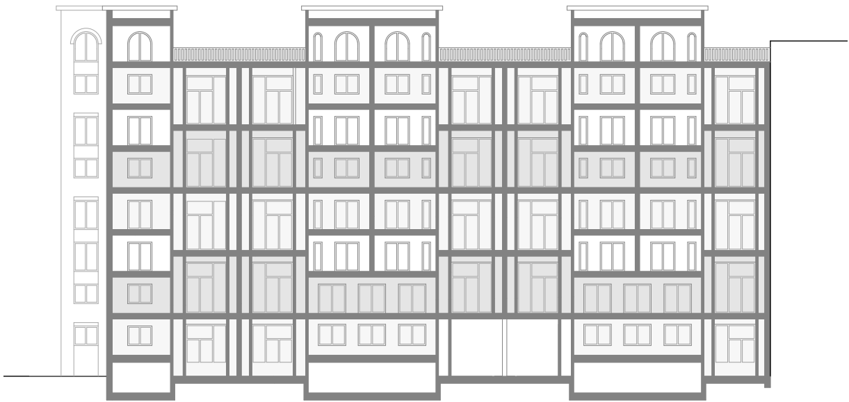
Schnitt A-A
