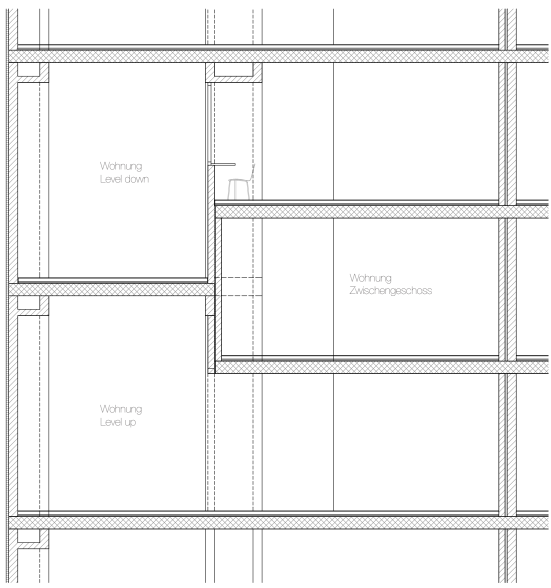
Schnitt C-C
