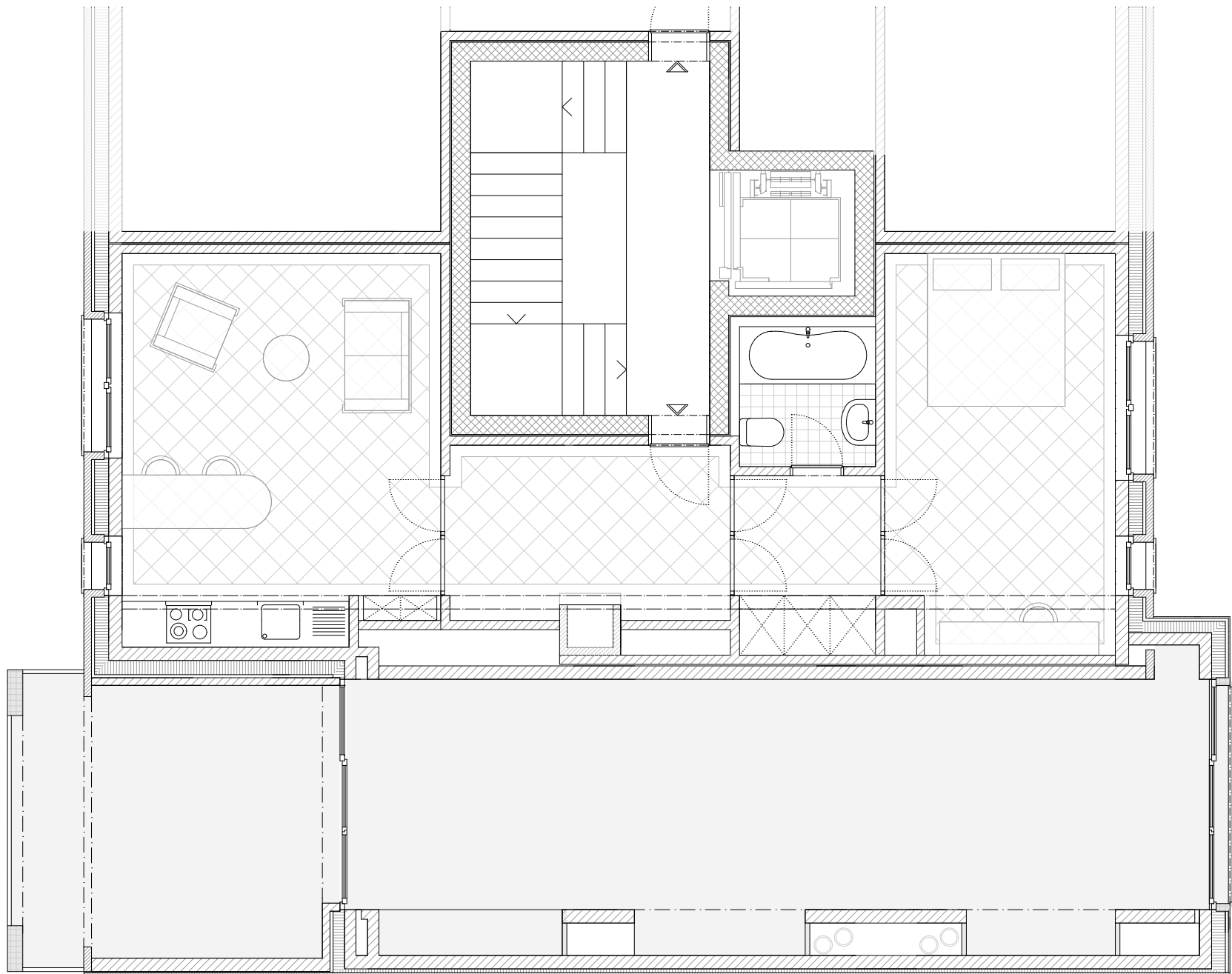
Grundriss Wohnung Level Down
