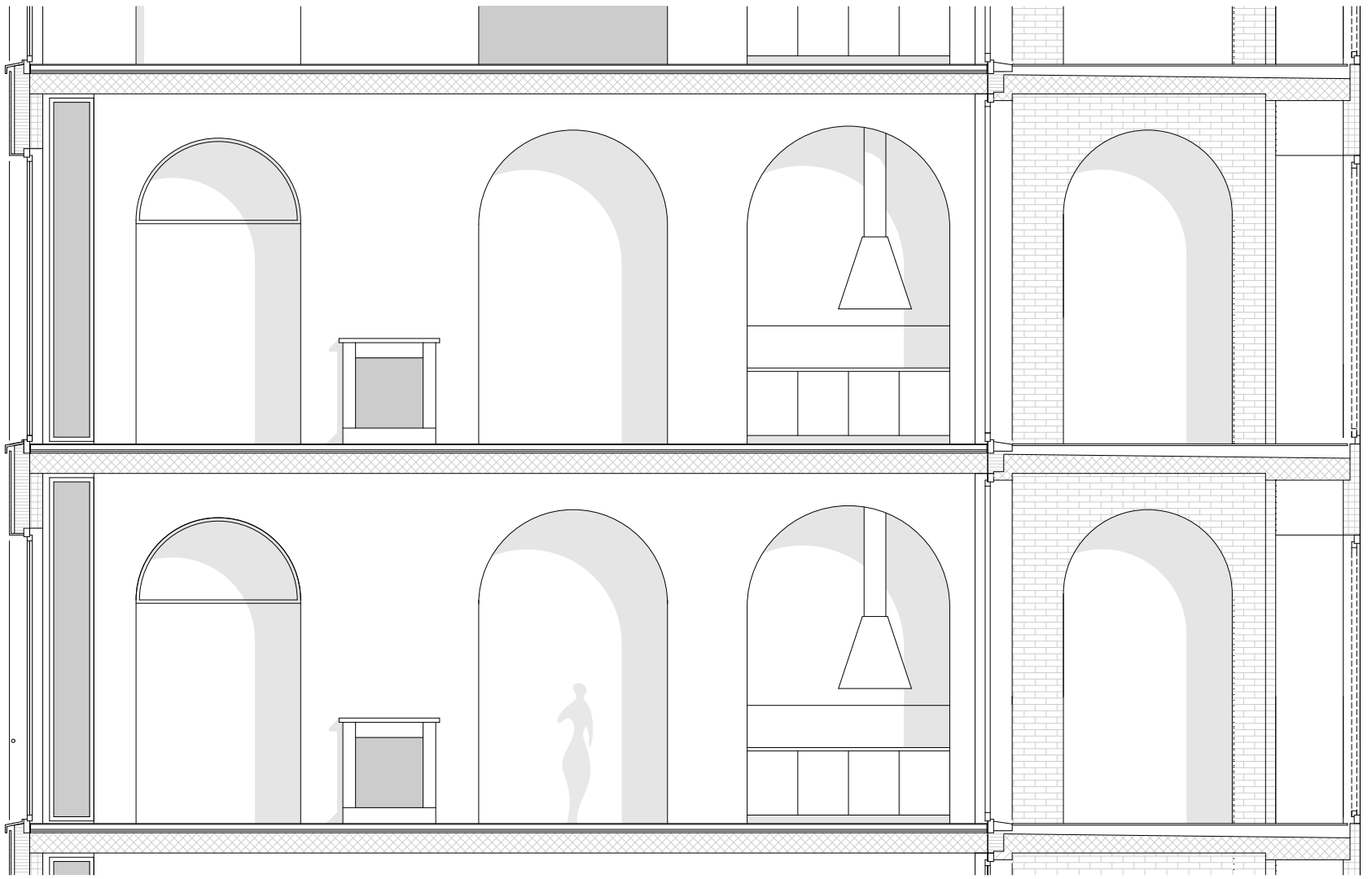
Schnitt B-B
